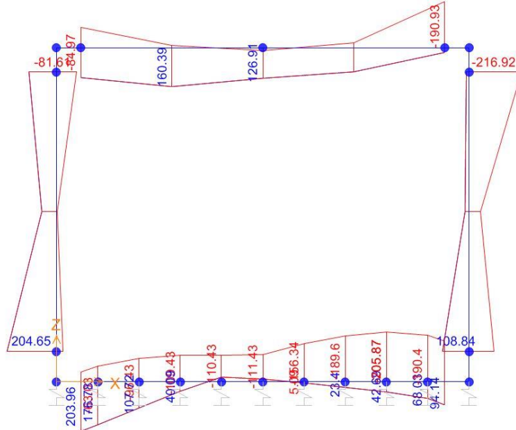
Momento Flettente
