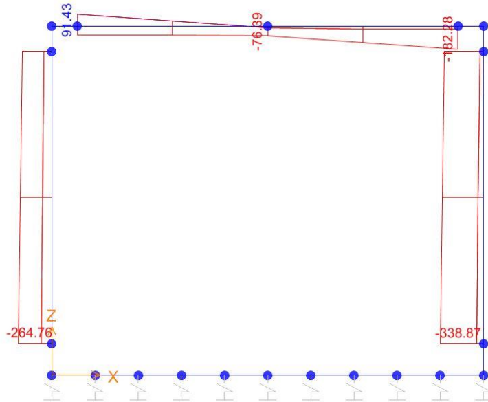
Sforzo normale
