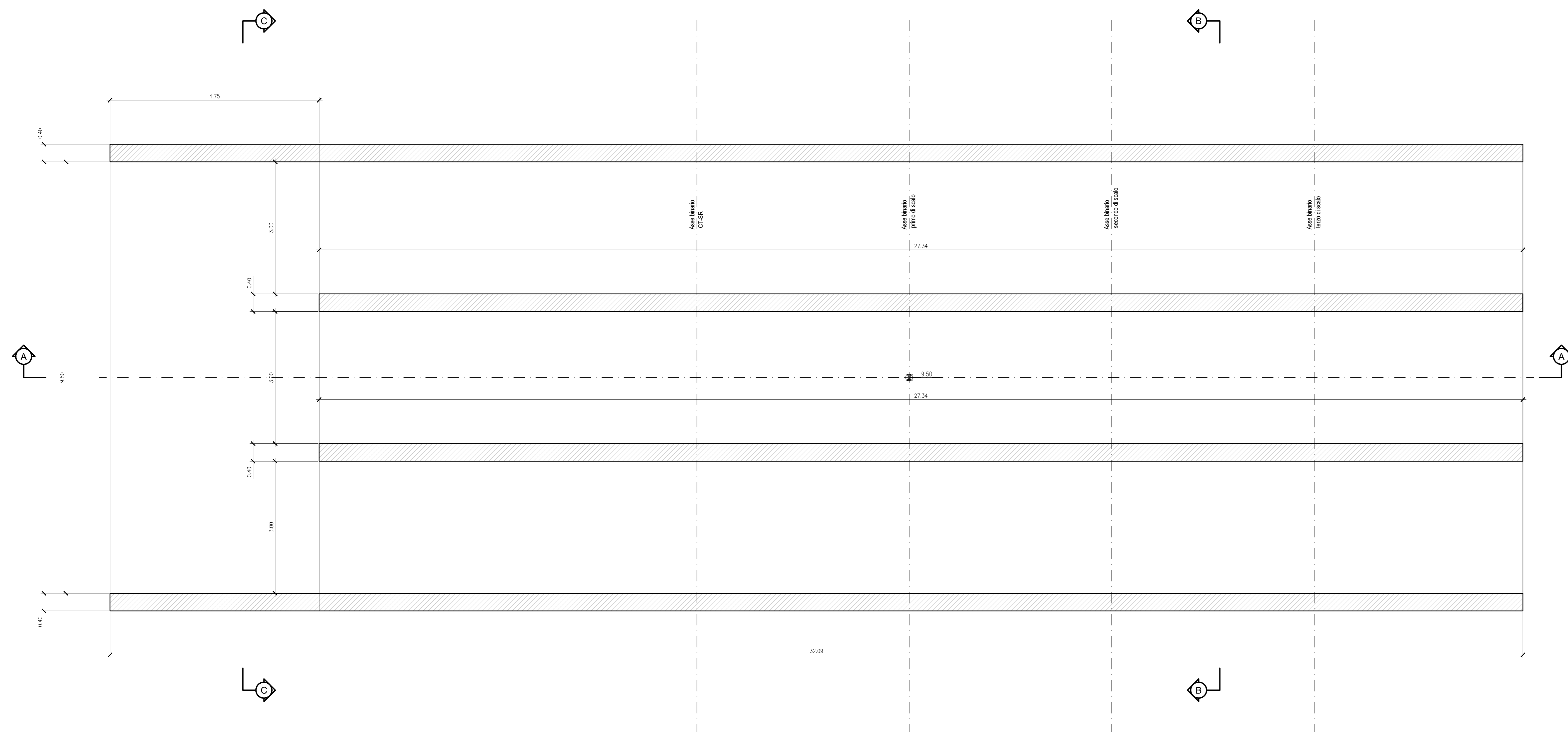
PIANTA SPICCATO IN12 SCALA 1:50
