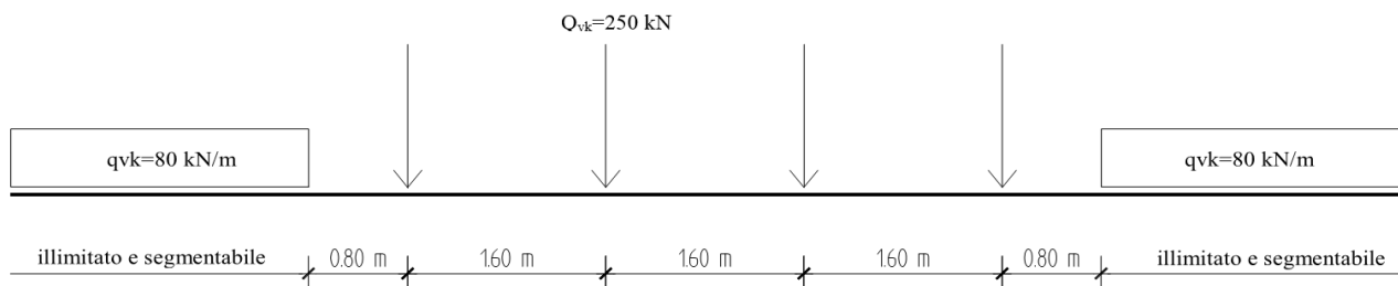
Figura 7. Treno LM71
