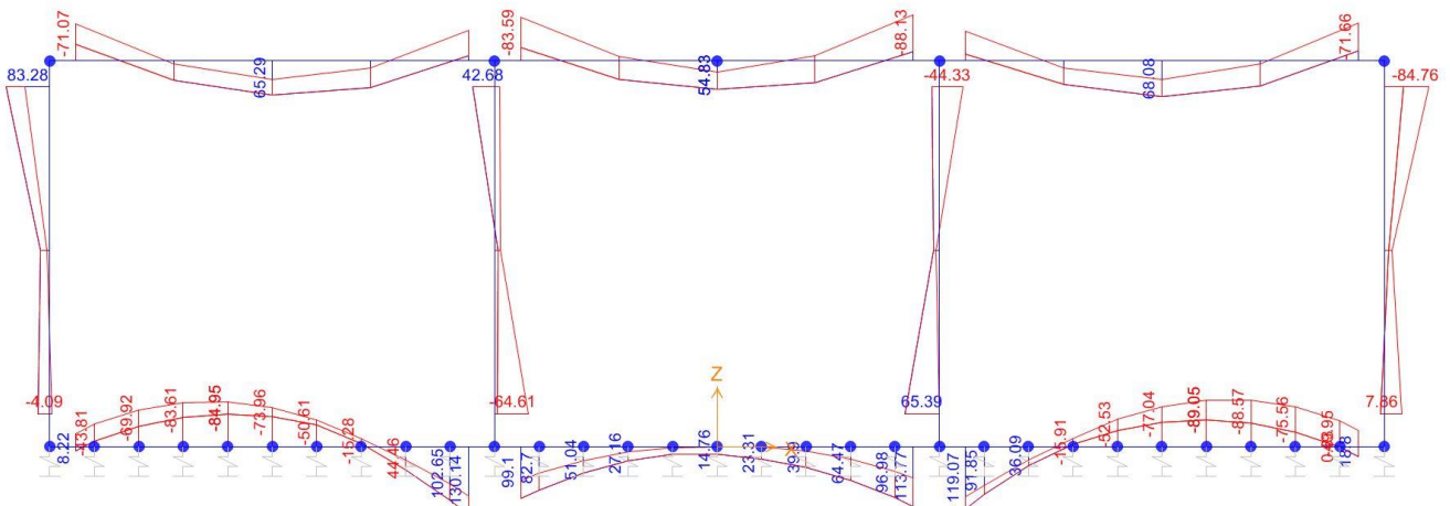
Momento Flettente
