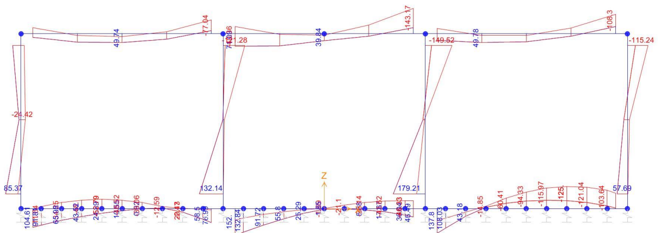
Momento Flettente
