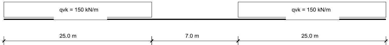
Figura 8. Treno SW/2
