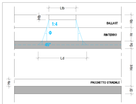
Figura 9. Schema modalità di diffusione dei carichi ferroviari
