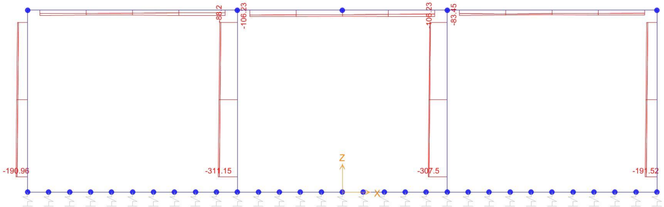
Sforzo normale
