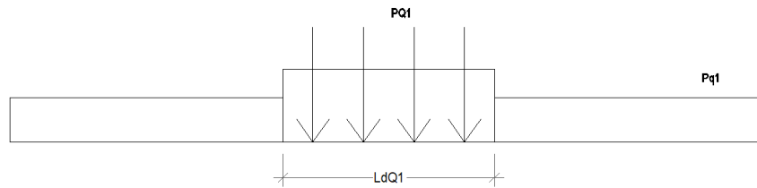
Figura 10. Carichi Treno LM71 su Ld
