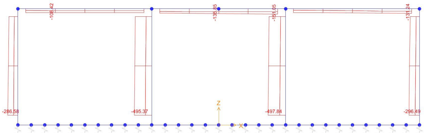
Diagrammi di involucro delle sollecitazioni: ENVELOPE SLU
