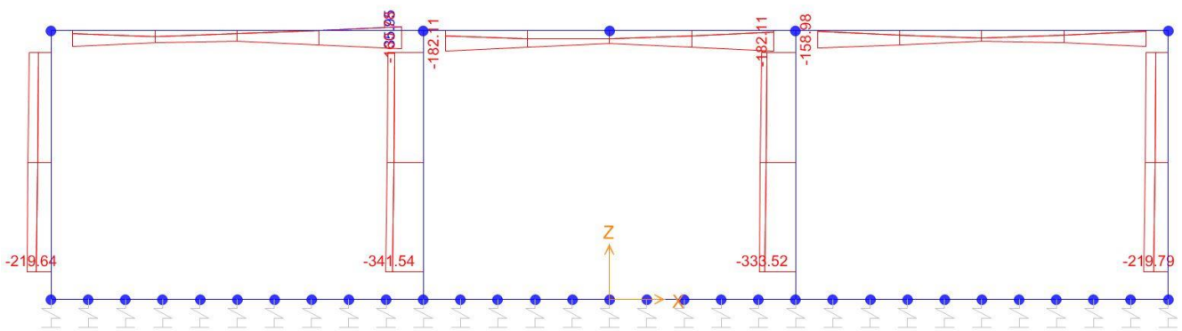
Sforzo normale
