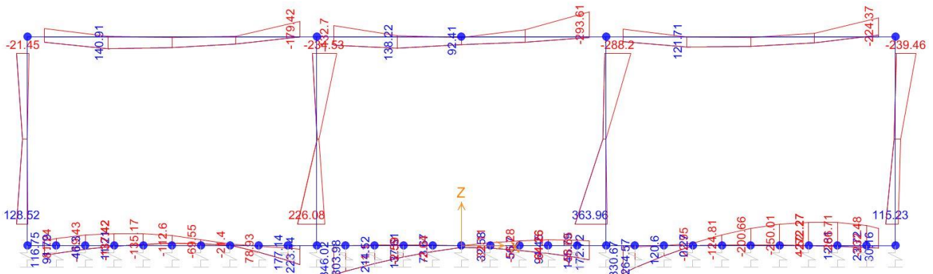
Momento Flettente
