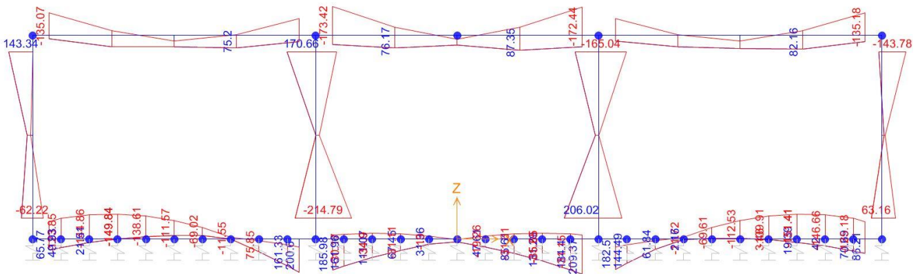
Momento Flettente
