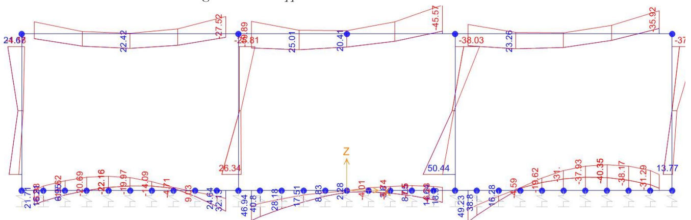
Diagrammi di involucro del momento: ENVELOPE SLV
