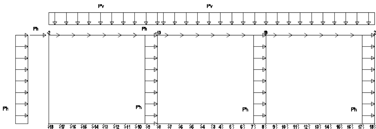
Figura 9. Forze sismiche agenti sulla struttura
