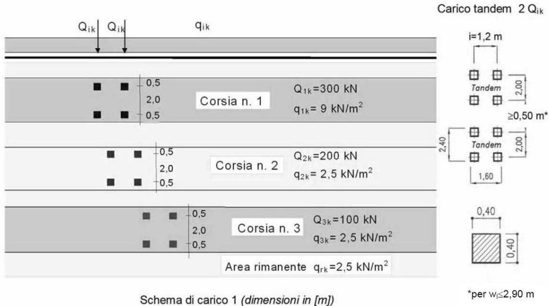
Figura 7 – Schema di Carico 1 del D.M. 17/01/2018
