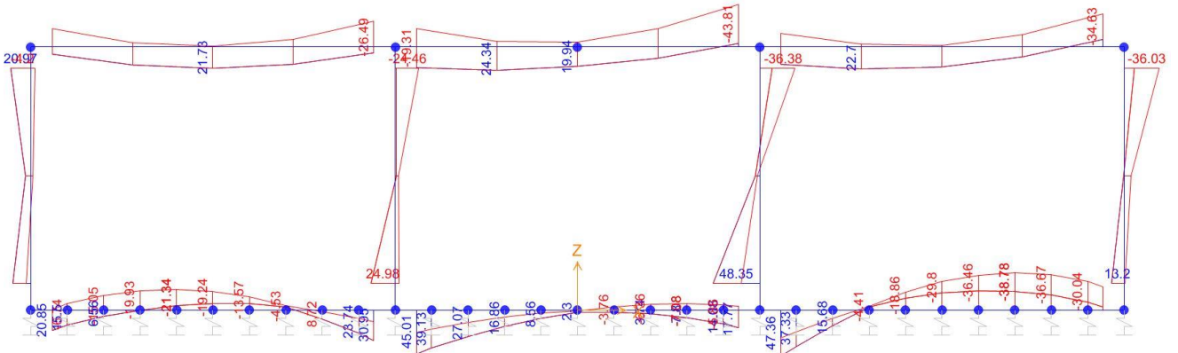
Diagrammi di involuppo del momento: ENVELOPE SLV
