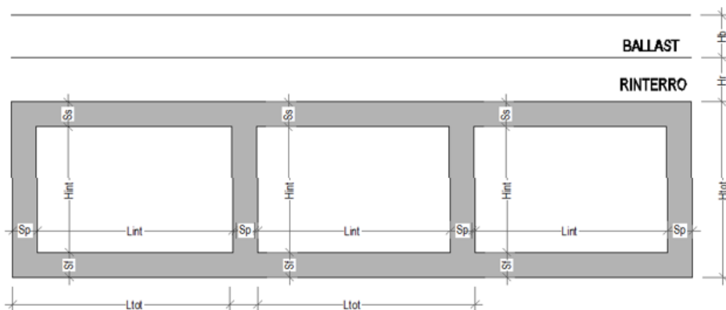
Figura 2. Sezione trasversale dello scatolare
