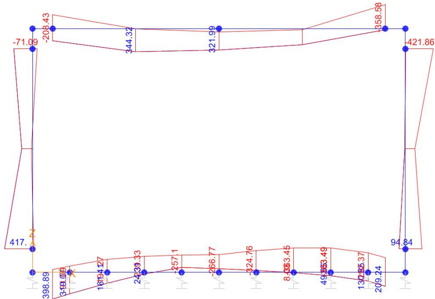
Momento Flettente
