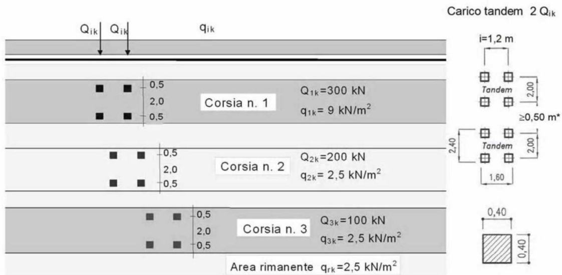
Figura 7 – Schema di Carico 1 del D.M. 17/01/2018
