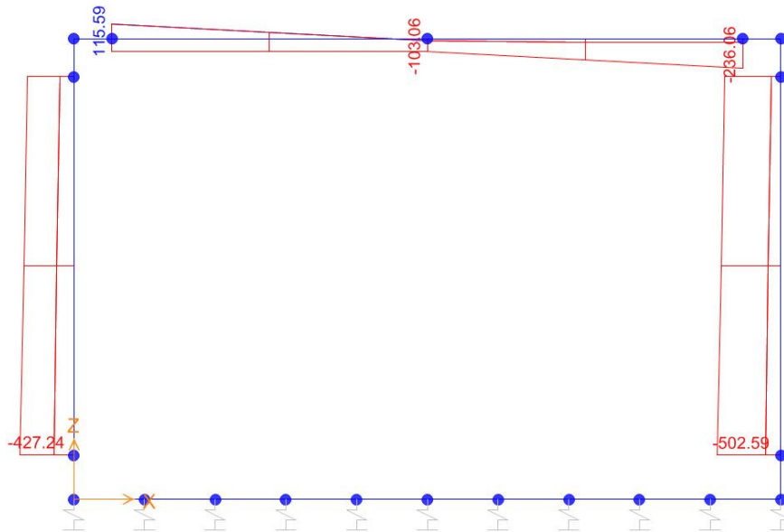
Sforzo normale
