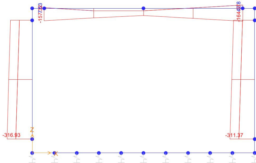
Sforzo normale
