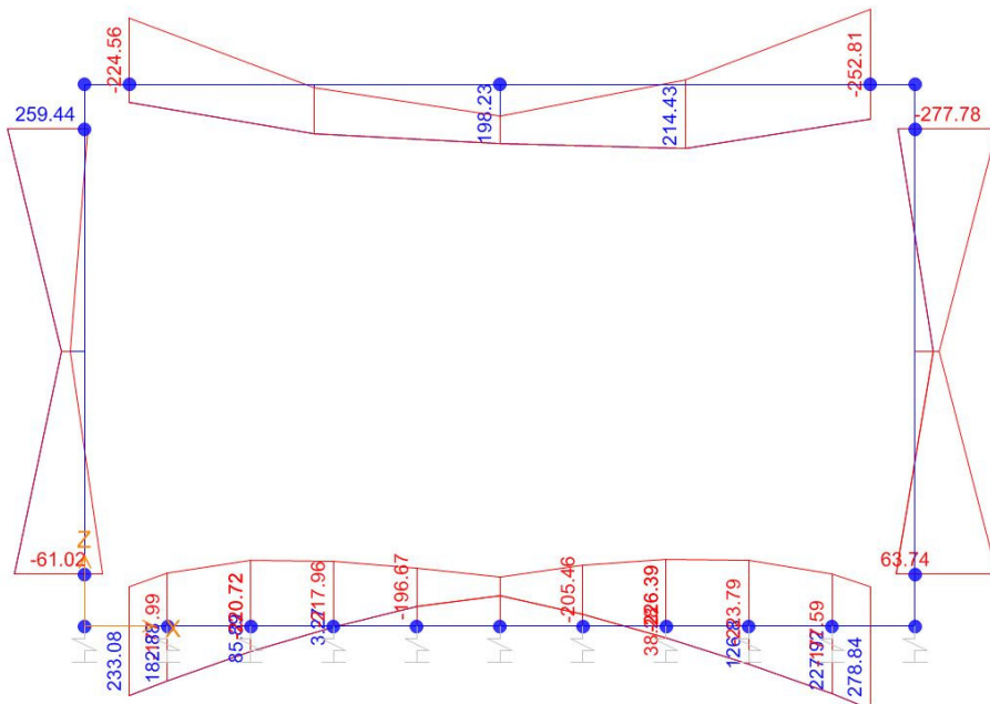
Momento Flettente
