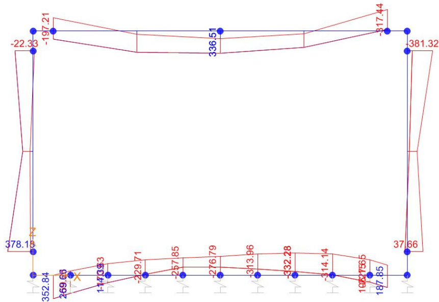
Momento Flettente
