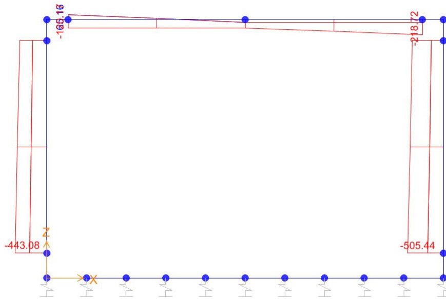
Sforzo normale
