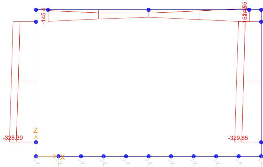
Sforzo normale
