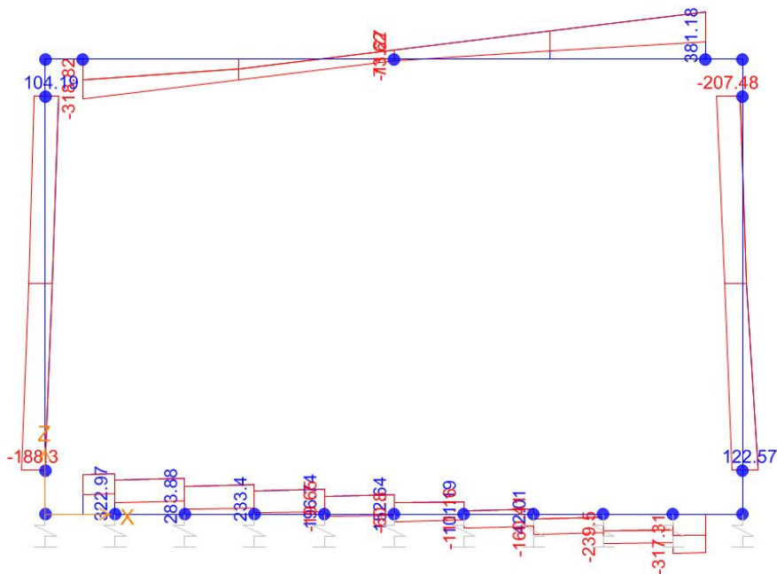
Taglio
