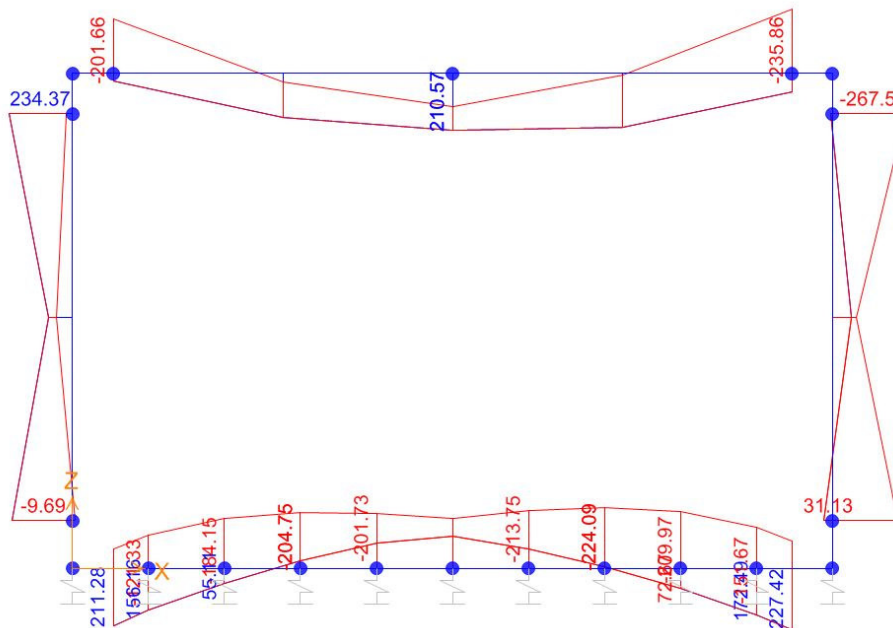
Momento Flettente
