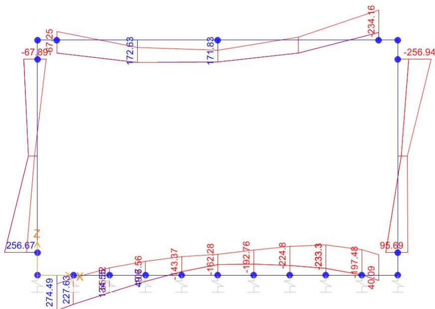
Momento Flettente
