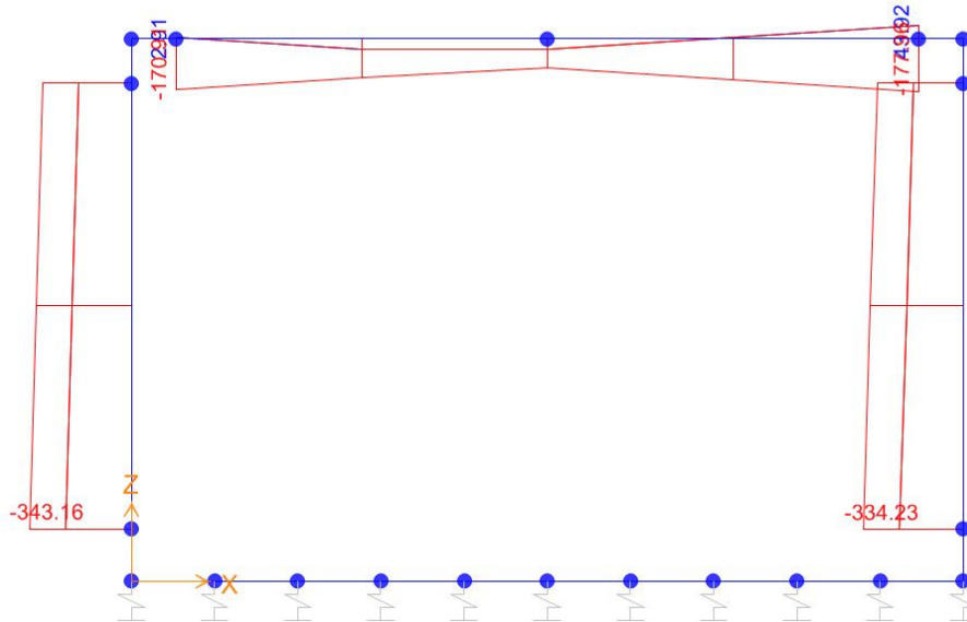
Sforzo normale
