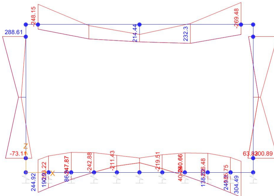
Momento Flettente
