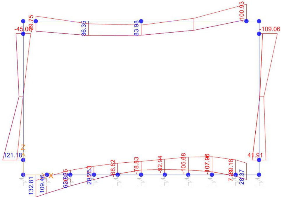
Momento Flettente
