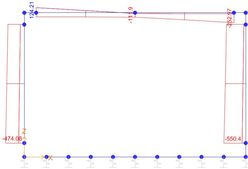
Sforzo normale
