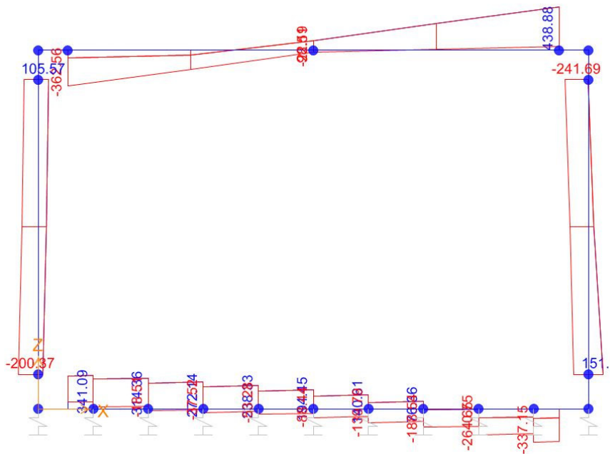
Taglio
