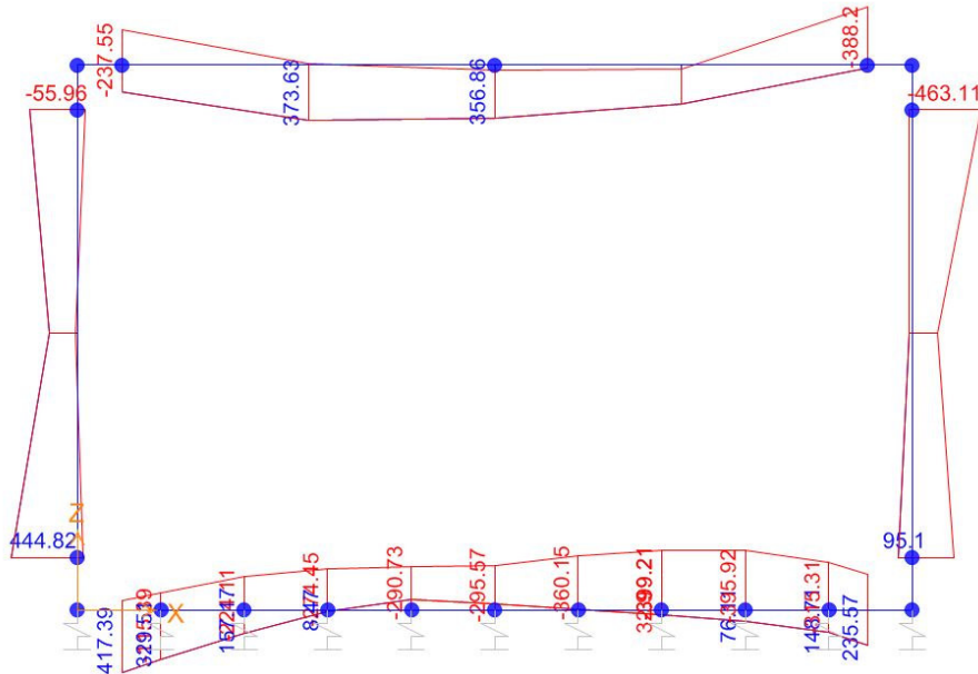
Momento Flettente
