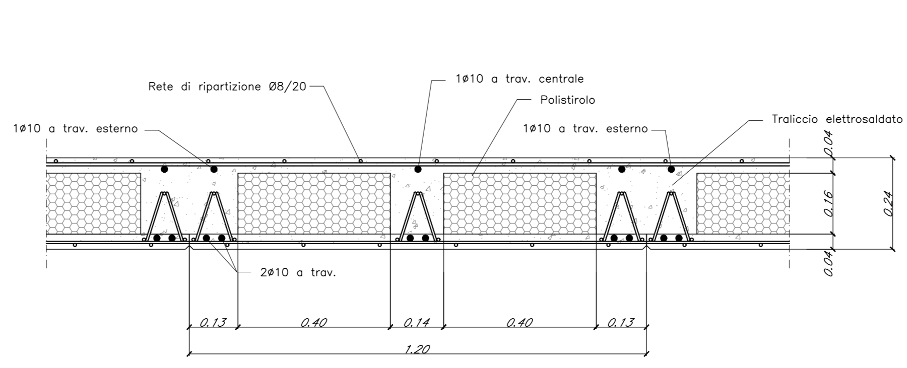
SEZIONE SOLAIO SCALA 1:10
