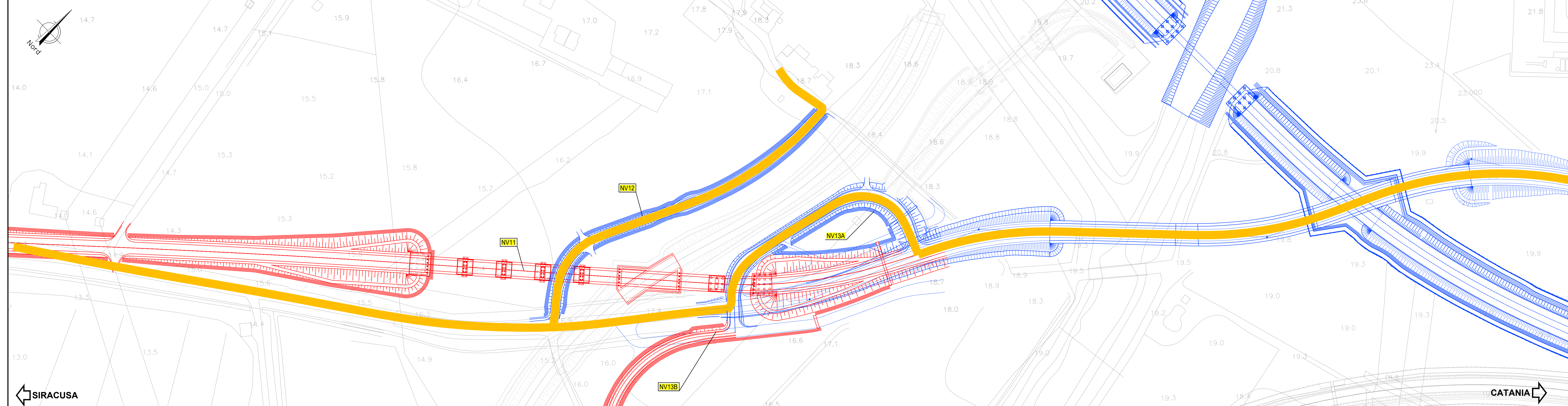
FASE 1 : TRAFFICO VEICOLARE DEVIATO SU NV13A E NV12 Demolizione tratto di viabilità' esistente con la NV11 Realizzazione della viabilità' NV11 e NV13B
