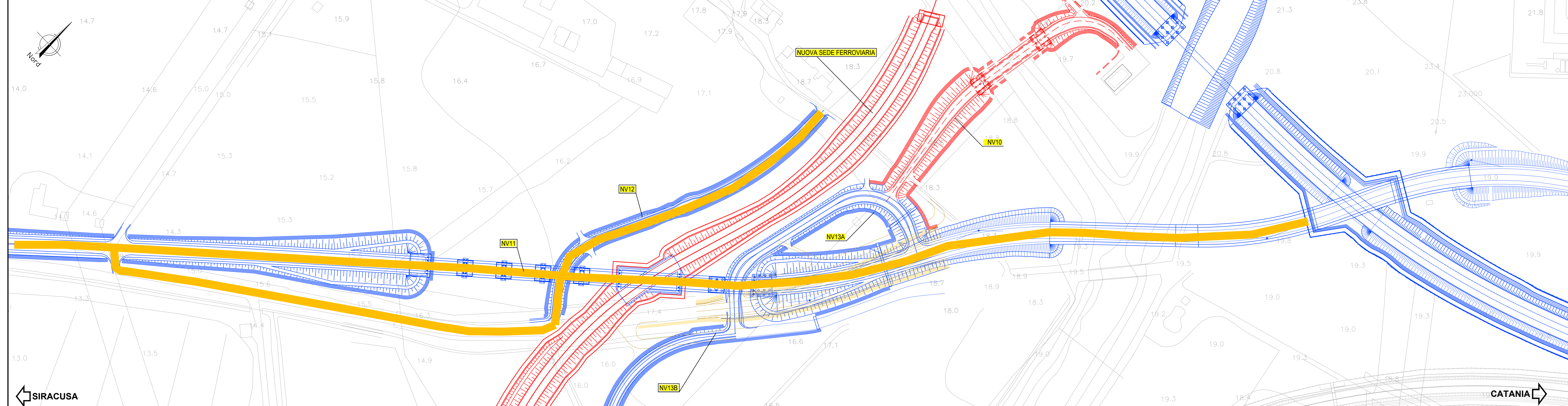
FASE 2 : TRAFFICO VEICOLARE DEVIATO SU NV11A E NV12 Apertura al traffico della nuova viabilità' NV11A Realizzazione della NV10 e della sede Ferroviaria
