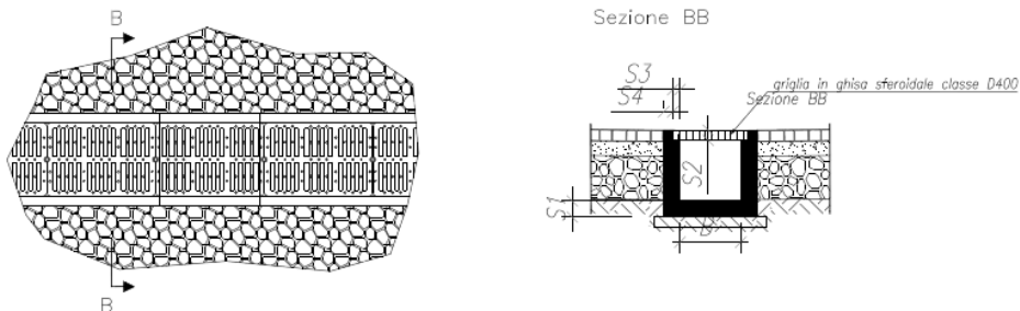
Figura 3-Tipologico canaletta grigliata
