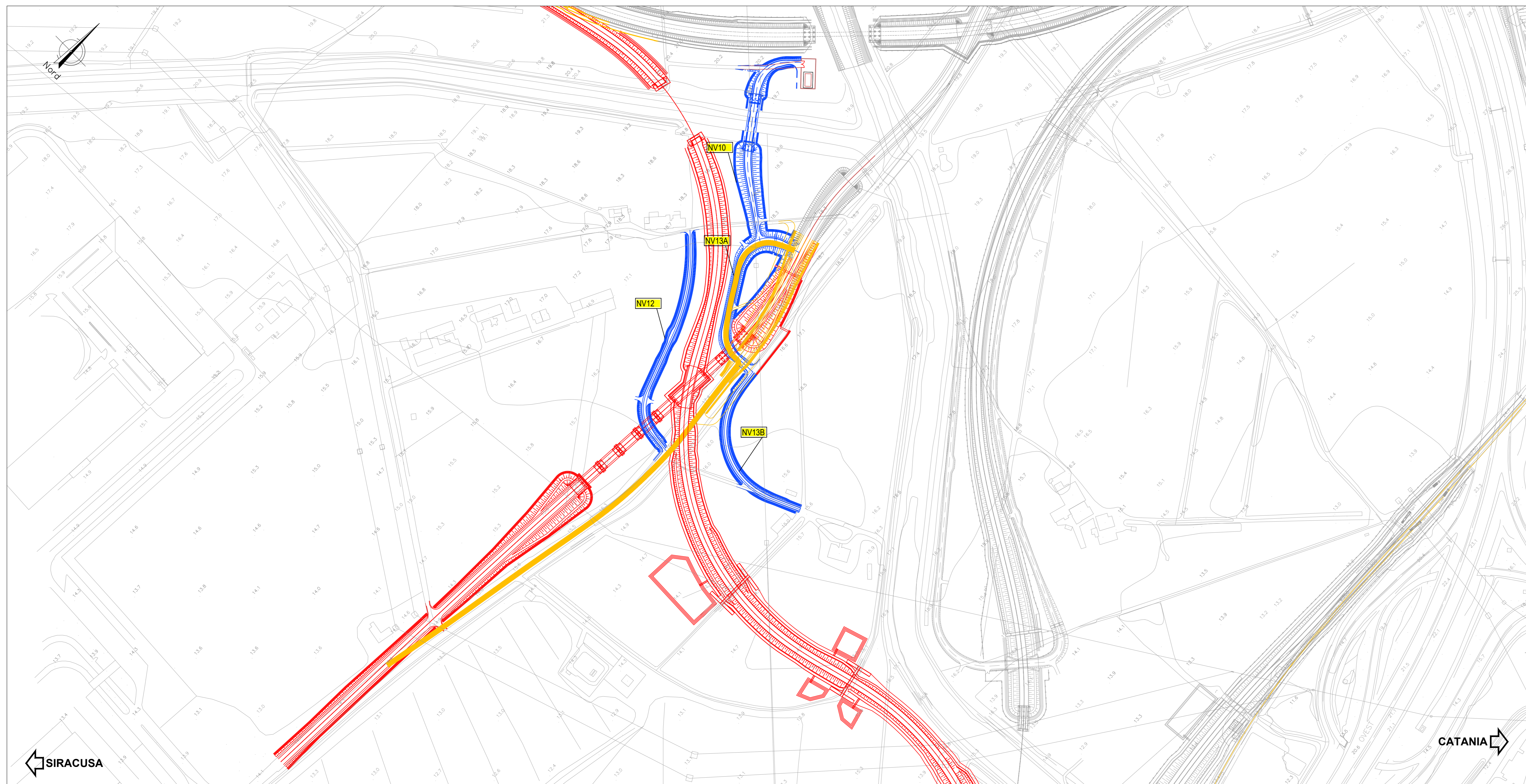
FASE 2 : TRAFFICO VEICOLARE SU SEDE NV13A In questa fase si prevede la demolizione del tratto NV12 PE Bicocca catenanuova interferente con la strada di progetto, per poi realizzare ed attivare la nuova NV11. Infine si prevede la realizzazione della linea ferroviaria.
