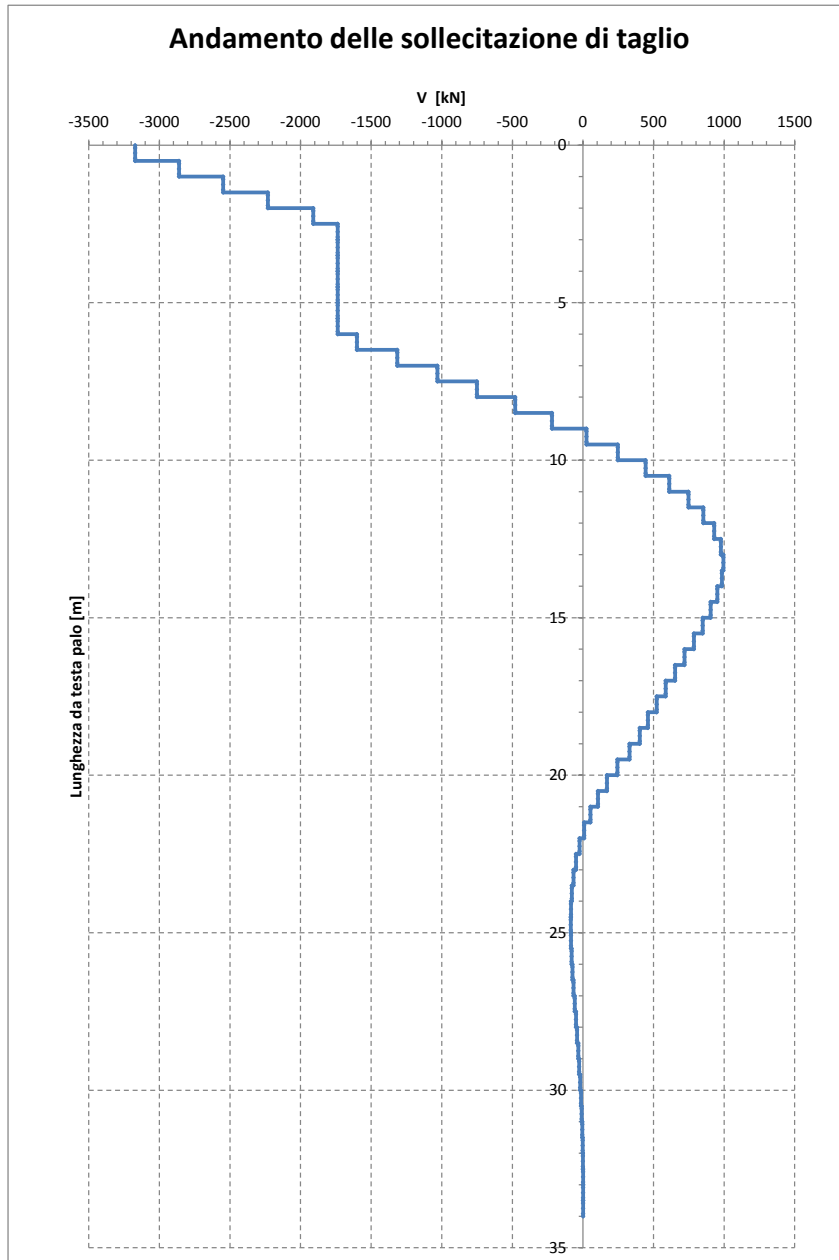
Figura 7 – Andamento del taglio lungo il palo - spalle NW03 NW04 con liquefazione
