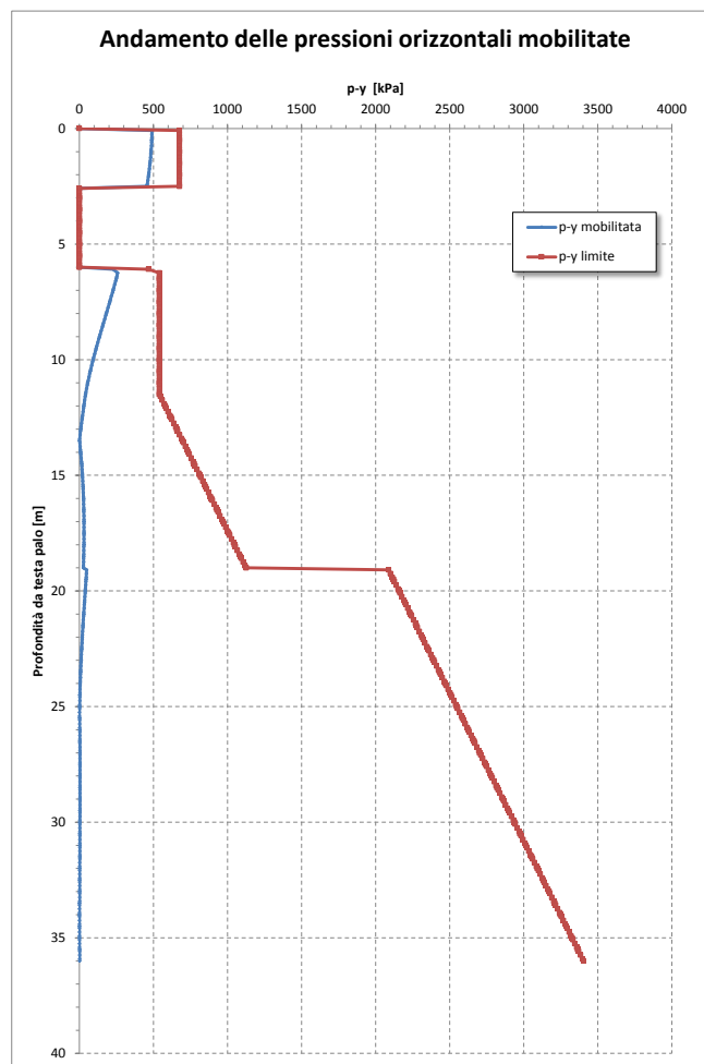
Figura 9 – Andamento pressioni orizzontali - pile NW03 NW04 con liquefazione
