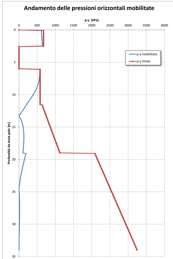
Figura 6 – Andamento pressioni orizzontali - spalle NW03 NW04 con liquefazione
