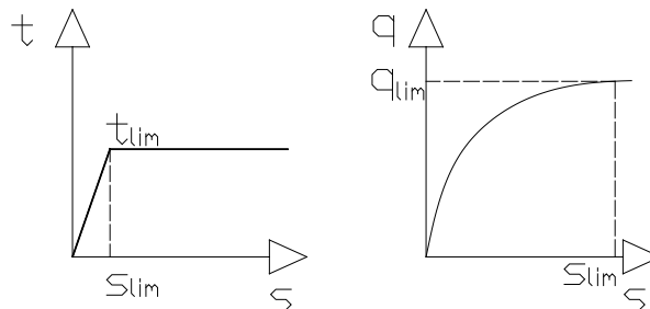
Figura 13 –curve di trasferimento (laterale e base)
