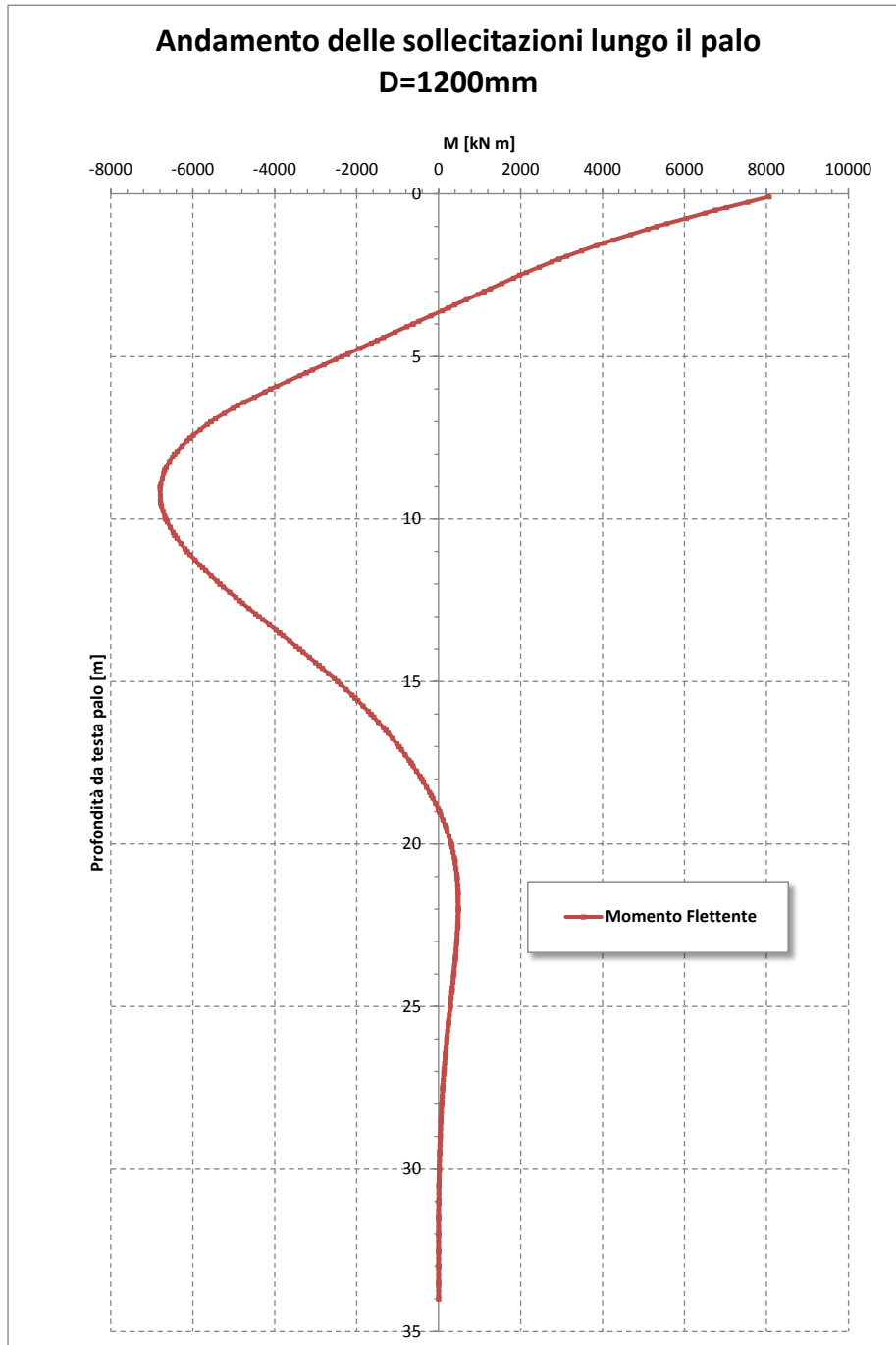
Figura 8 – Andamento del momento lungo il palo – spalle NW03 NW04 con liquefazione
