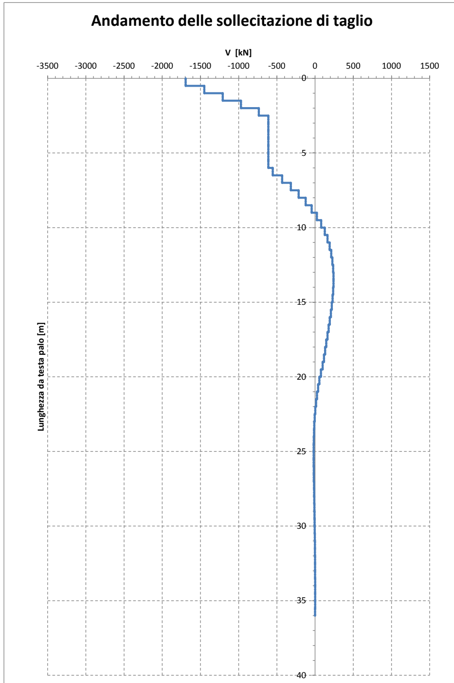
Figura 10 – Andamento del taglio lungo il palo – pile NW03 NW04 con liquefazione
