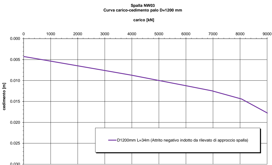
Figura 17 –curva carico-cedimento singolo palo in presenza di attrito negativo indotto dal rilevato di appoggio alla spalla – D=1200 mm
