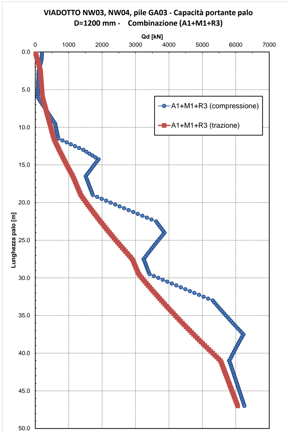
Figura 2 – Portata di progetto – in presenza di liquefazione
