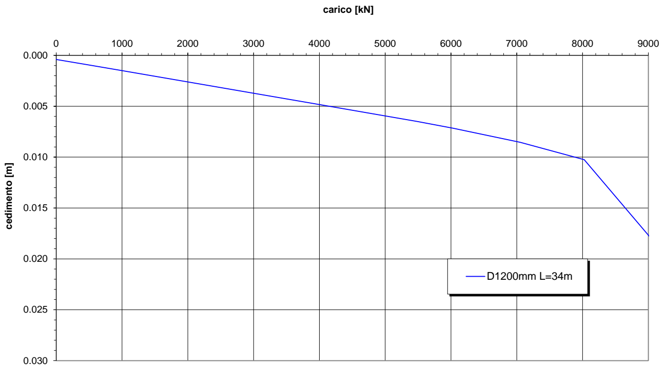
Figura 15 –curva carico-cedimento singolo palo in presenza di potenziale liquefazione – D=1200 mm
