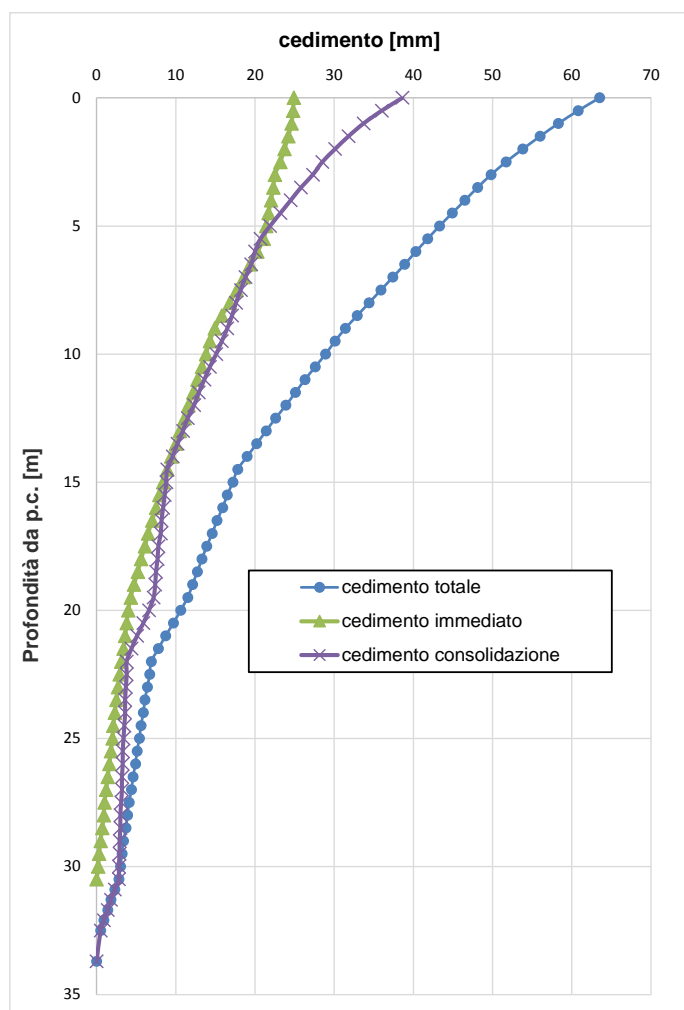
Figura 16 – Cedimento totale indotto dal rilevato di approccio alla spalla D del NW03
