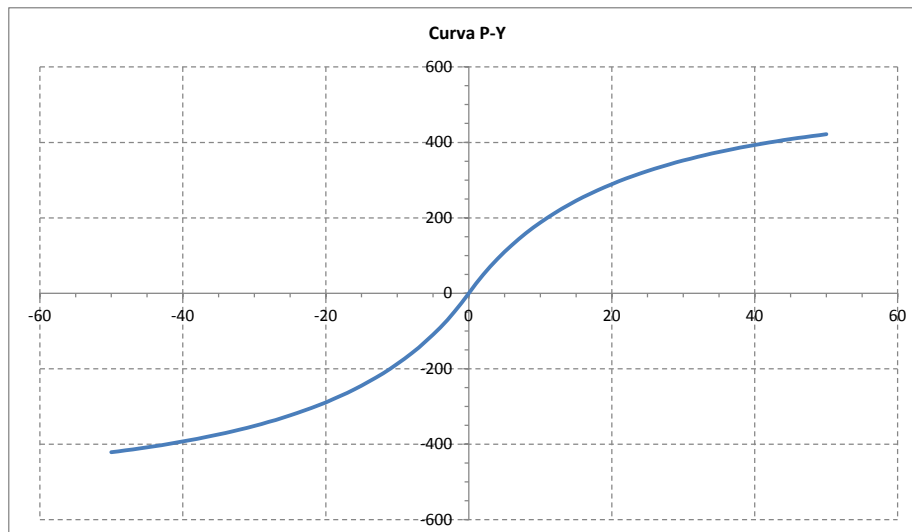
Figura 5 – curva P-Y a quota 8 m da testa palo – NW03-NW04 con liquefazione
