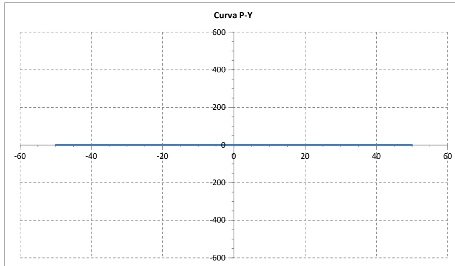
Figura 4 – curva P-Y a quota 5.0 m da testa palo – NW03-NW04 con liquefazione (strato liquefacibile, reazione nulla)
