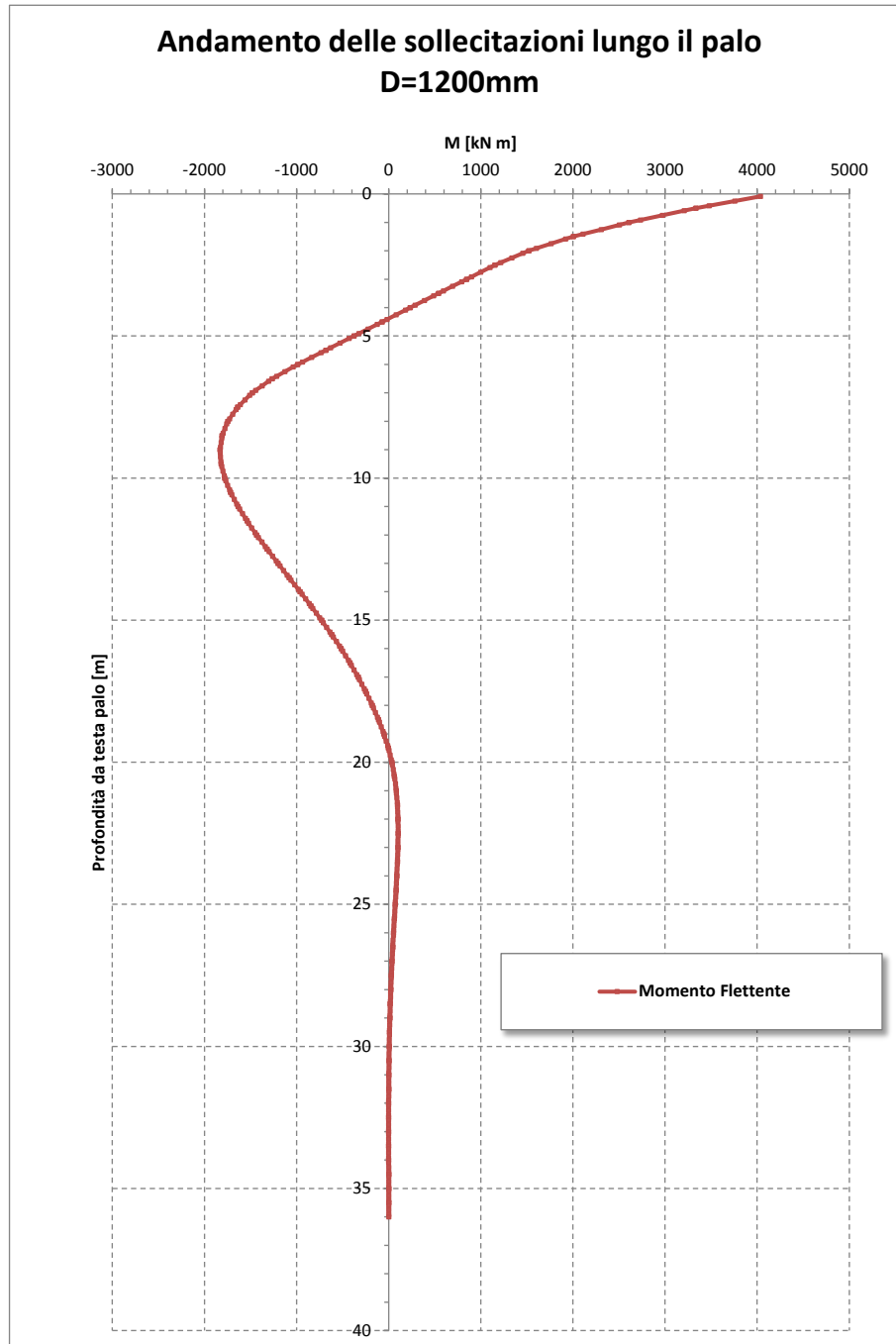
Figura 11 – Andamento del momento lungo il palo - pile NW03 NW04 con liquefazione
