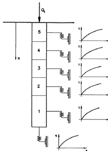
Figura 12 –Legame ideale palo-terreno
