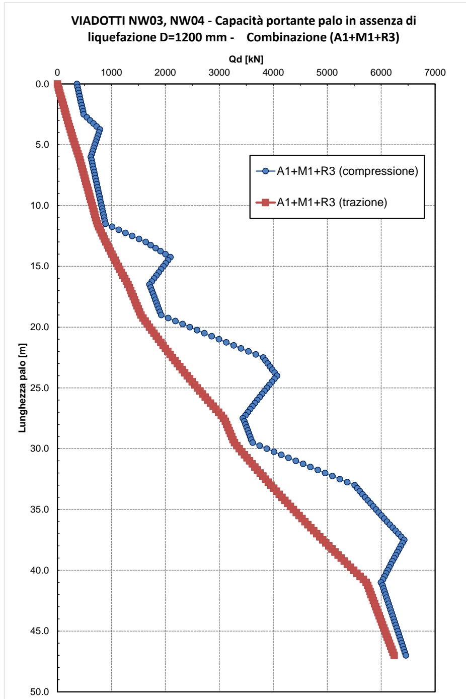
Figura 3 – Portata di progetto – in assenza di liquefazione
