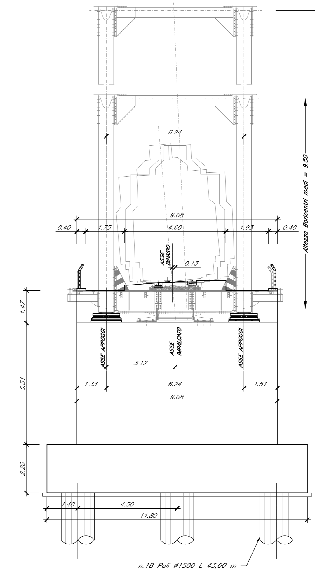
SEZIONE TRASVERSALE Scala 1:100
