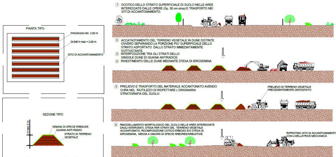
Figura 6-1: Schema di accantonamento del terreno vegetale
