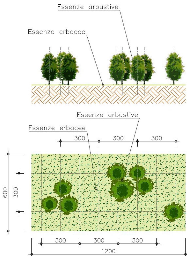
Figura 4 – Modulo C – Sistemazione spondale
