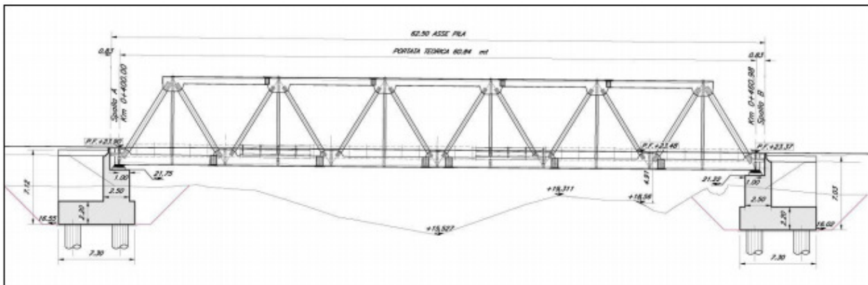
Figura 6 Sezione longitudinale dell'impalcato
