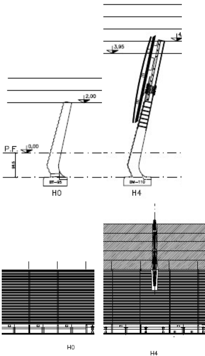
Sezioni-tipo dei moduli di barriera antirumore previsti nello Studio Acustico
