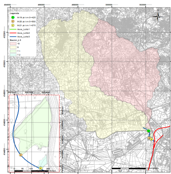
Inquadramento dei bacini idrografici ricadenti nel lotto 3
