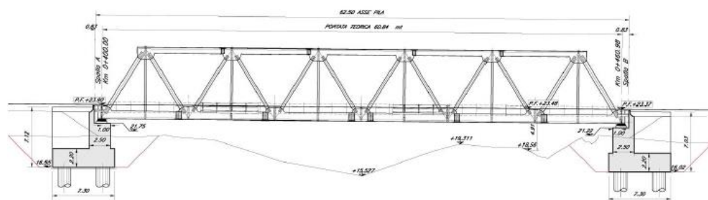
Sezione longitudinale dell'impalcato
