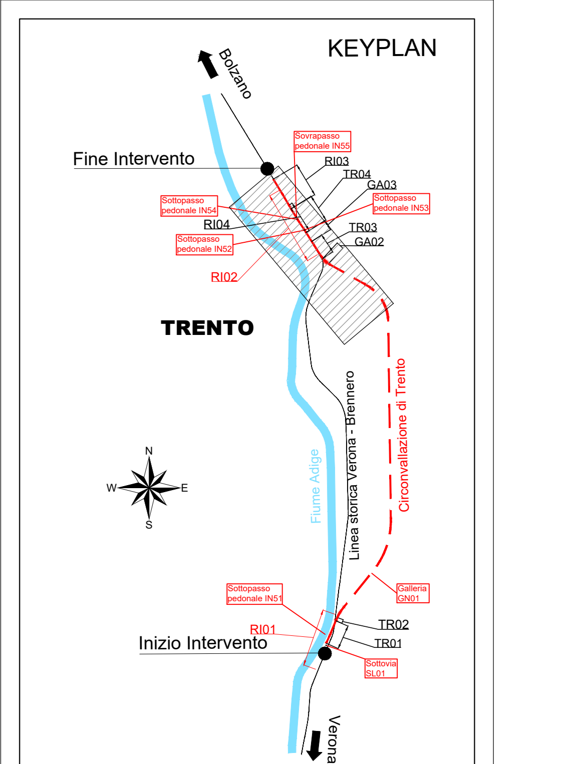
PLANIMETRIA DI PROGETTO VARIANTE LINEA STORICA LOCALITA' SCALO FILZI Scala 1:2000
