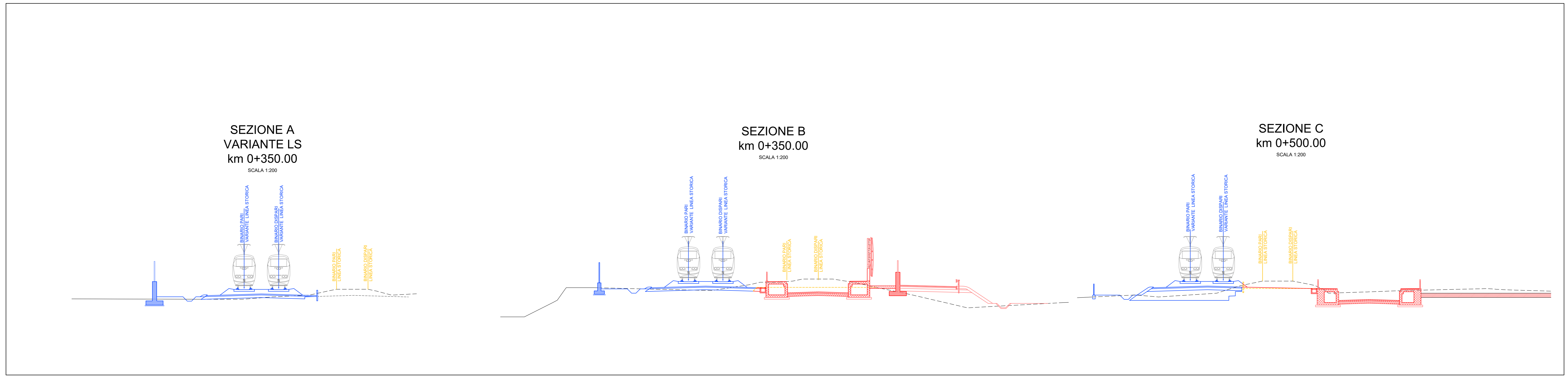
ZONA ACQUAVIVA SEZIONI ILLUSTRATIVE MACROFASE 2a SCALA 1:200
