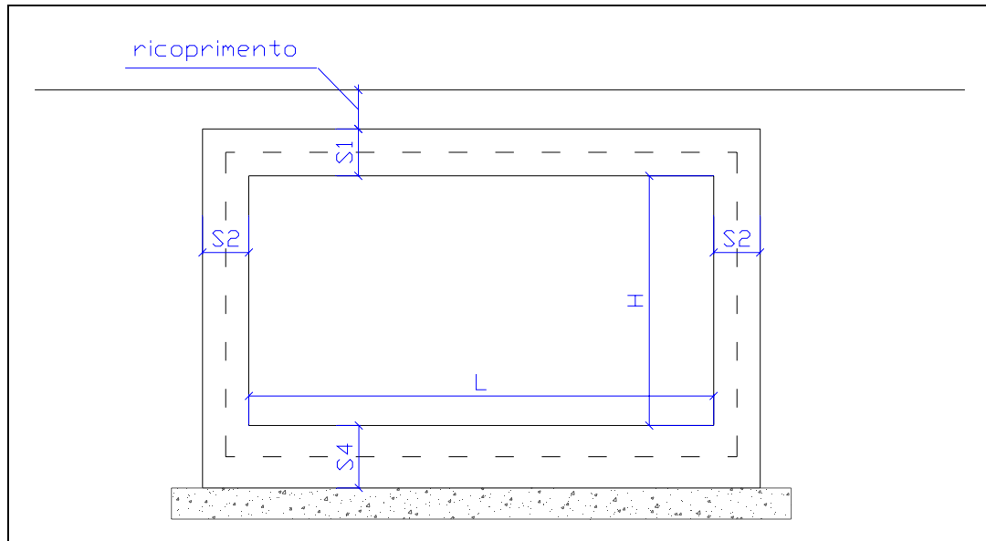
Figura 4-1 – Geometria della struttura
