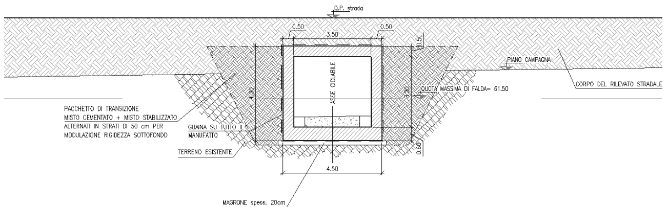
Figura 1-1 - Sezione trasversale
