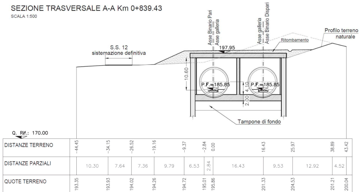
Figura 2. Imbocco sud
