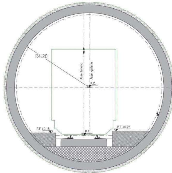
Figura 1. Profilo di intradosso galleria a doppia canna
