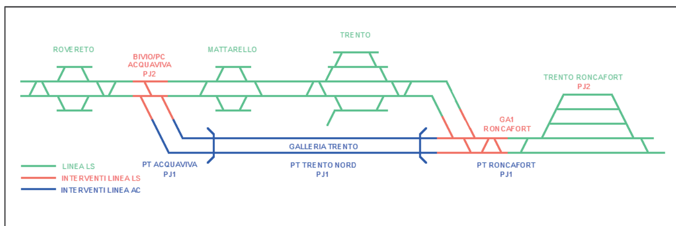
Figura 1: schema funzionale Lotto 3
