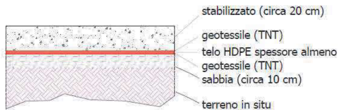
Figura 5 Tipologico Capping per aree di cantiere poste presso siti contaminati
