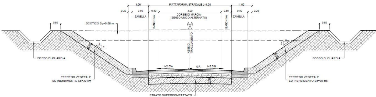
Figure 6-2: Dest. Particolare 6 m - sezione tipo in rilevato H_{rail} > 6.00 m
