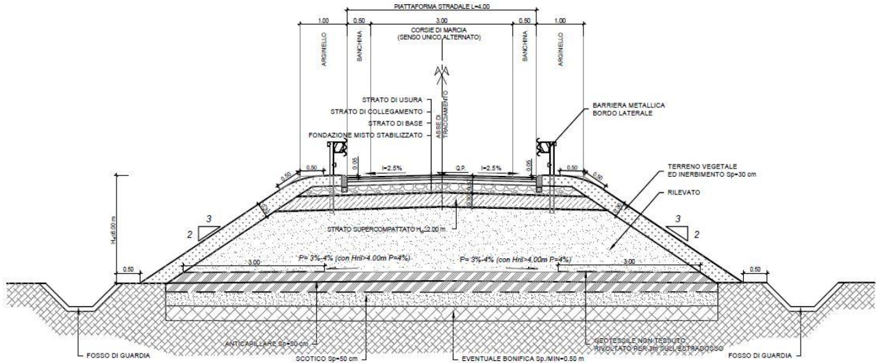
Figure 6-1: Dest. Particolare 6 m - sezione tipo in rilevato H_{rail} \leq 6.00 m
