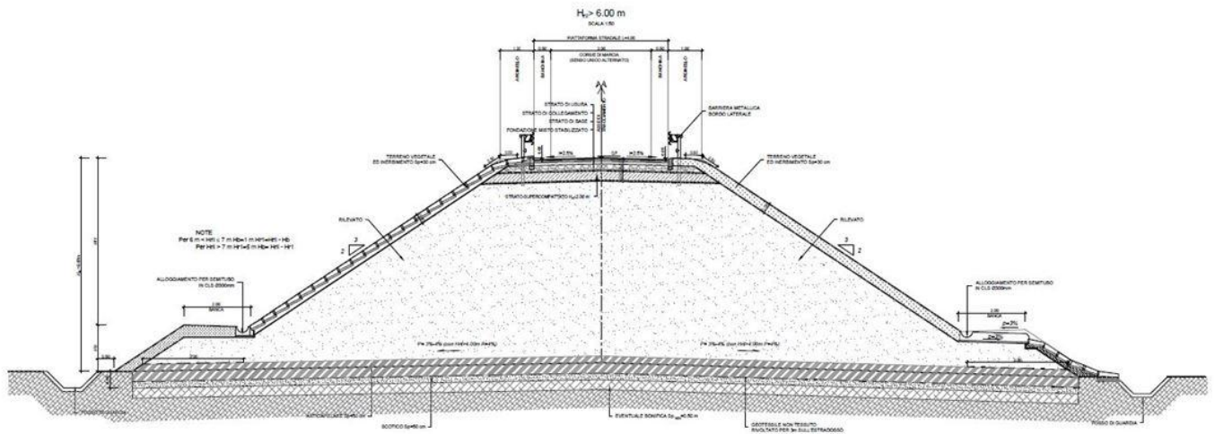
Figure 6-3: Dest. Particolare 6 m - sezione tipo in trincea
