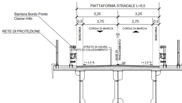
Figure 6-4: Dest. Particolare 6.5m - sezione tipo in viadotto
