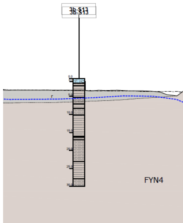
Figura 2. Profilo geologico
