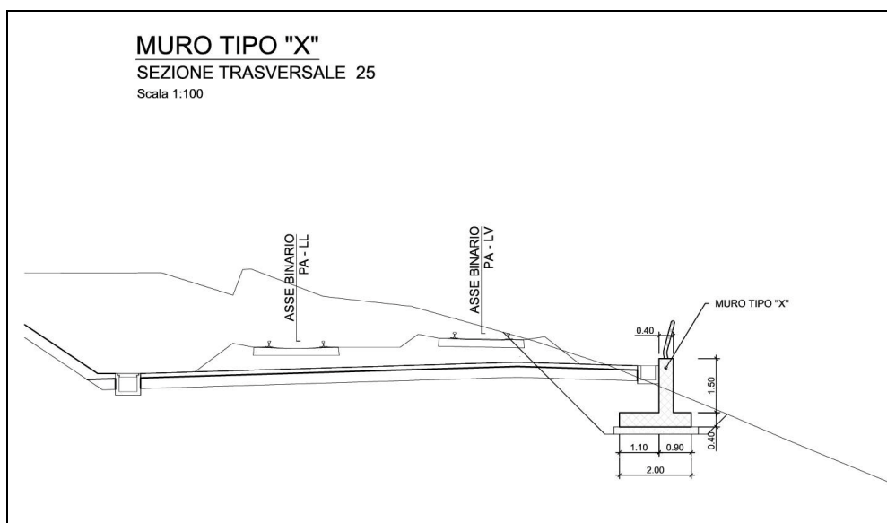
Figura 1-3 – TR02 - RI01: Muro di sostegno MU02 – Sezione tipo X.
