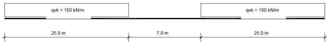
Figura 8-10 – Treno di carico SW2.
