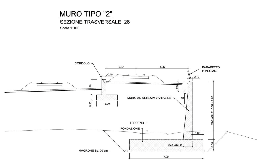
Figura 1-5 – TR02 - RI01: Muro di sostegno MU02 – Sezione tipo 2.
