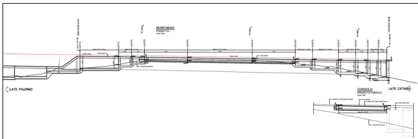
Figura 1-2 – TR02 - RI01: Muro di sostegno MU02 - Prospetto.
