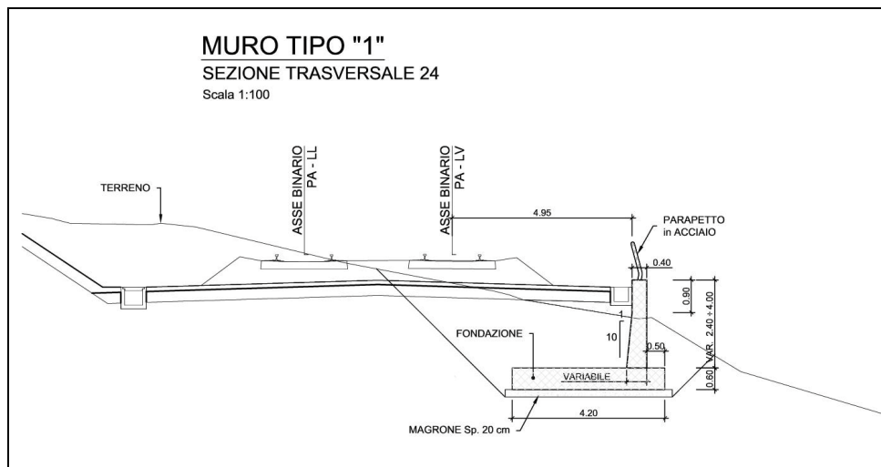
Figura 1-4 – TR02 - RI01: Muro di sostegno MU02 – Sezione tipo 1.
