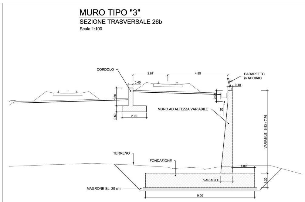
Figura 1-6 – TR02 - RI01: Muro di sostegno MU02 – Sezione tipo 3.
