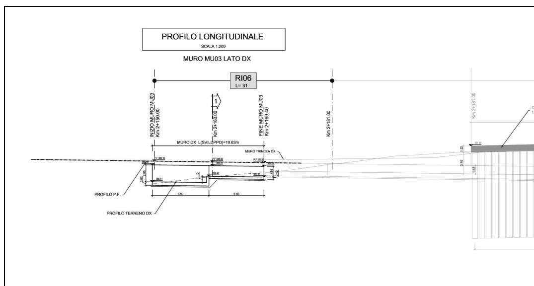
Figura 1-2 – RI06: Muri di sostegno MU03 – Prospetto tipo 0.
