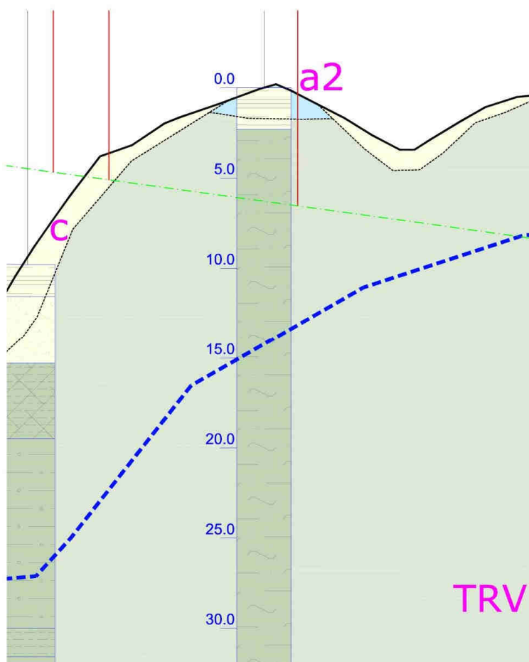
Figura 6-1 – Stralcio del profilo geotecnico.
