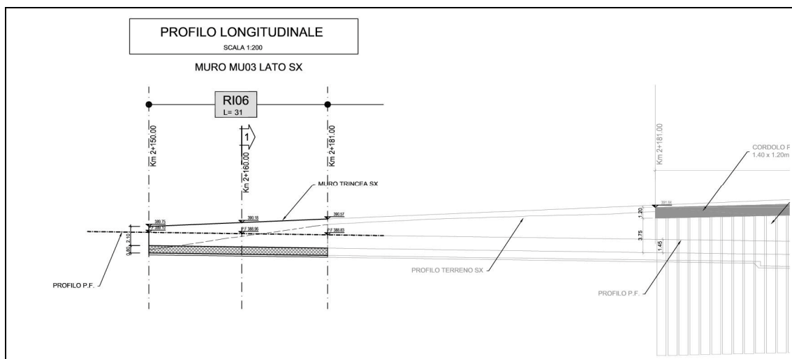
Figura 1-3 – RI06: Muri di sostegno MU03 – Prospetto tipo 1.
