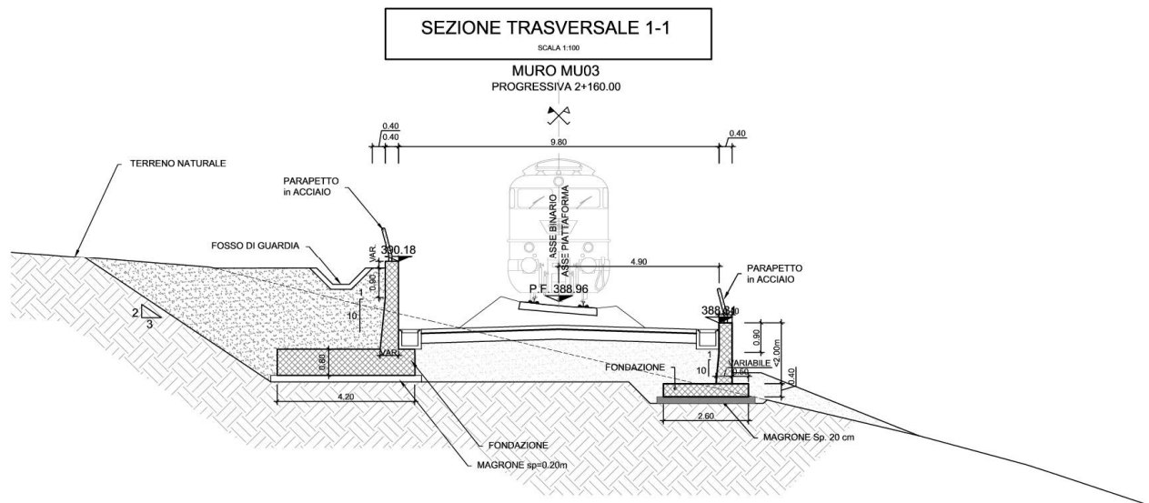
Figura 1-4 – RI06: Muri di sostegno MU03 – sezione tipo 0 e 1.
