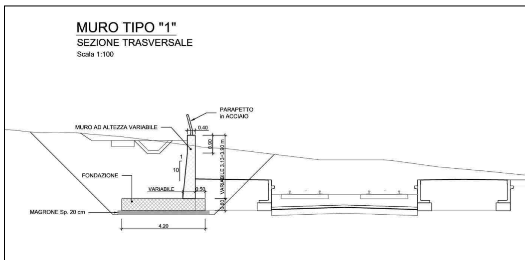
Figura 1-5 – TR12: Muro di sostegno MU02 – Sezione tipo 3.
