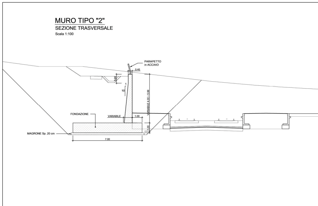
Figura 1-4 – TR12: Muro di sostegno MU02 – Sezione tipo 2.
