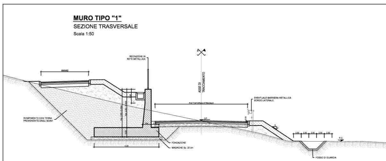
Figura 1-3 – NV04E: Muro di sostegno MU15A - Sezione.
