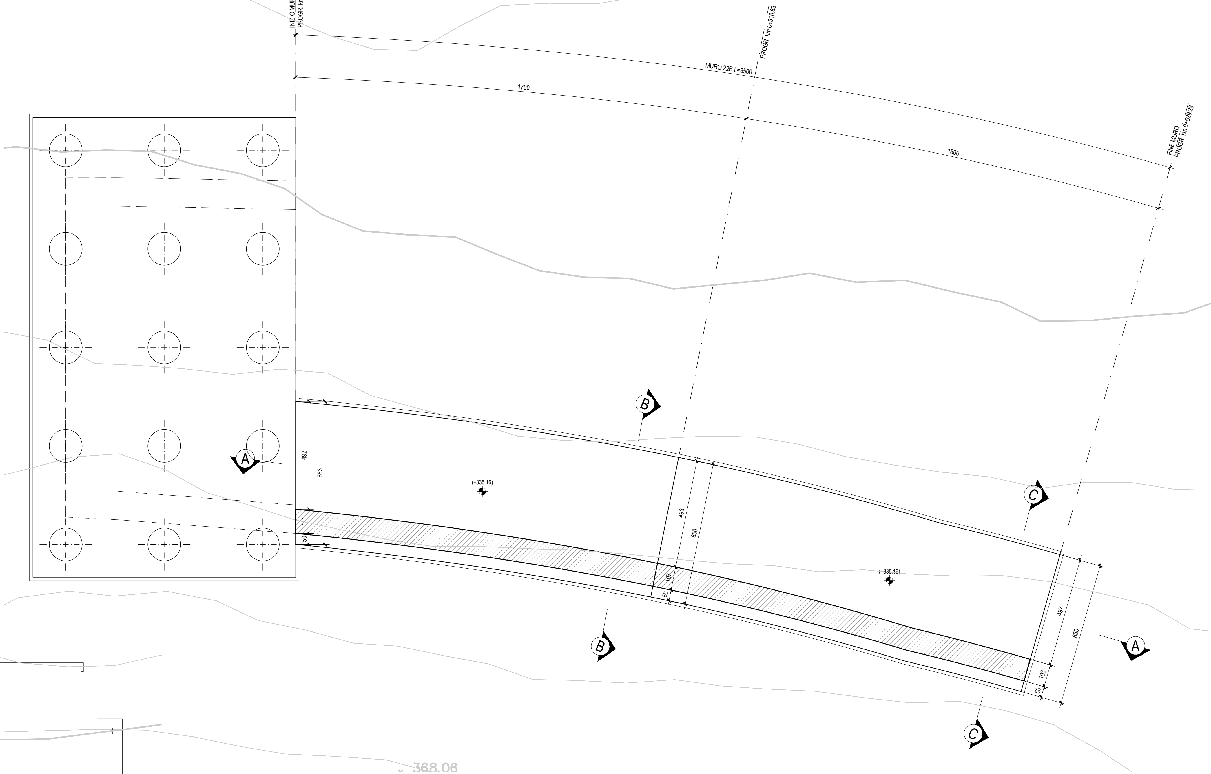
PIANTA SPICCATO - Scala 1:100
