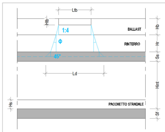
Figura 9. Schema modalità di diffusione dei carichi ferroviari
