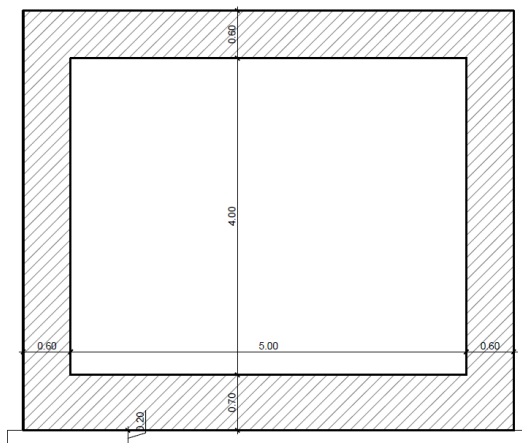
Figura 1c. Sezione trasversale dello scatolare
