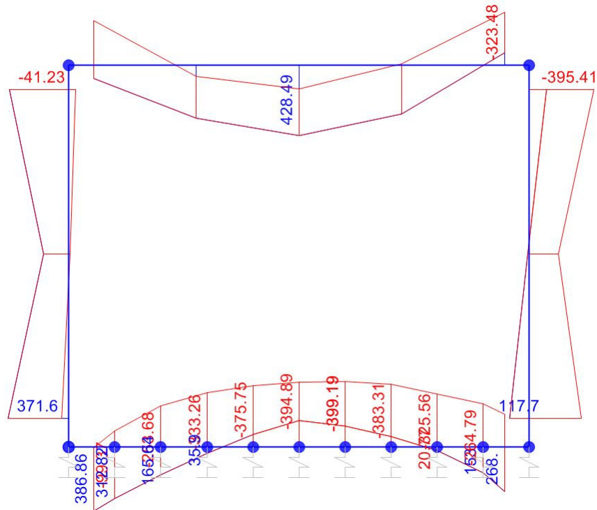
Momento Flettente
