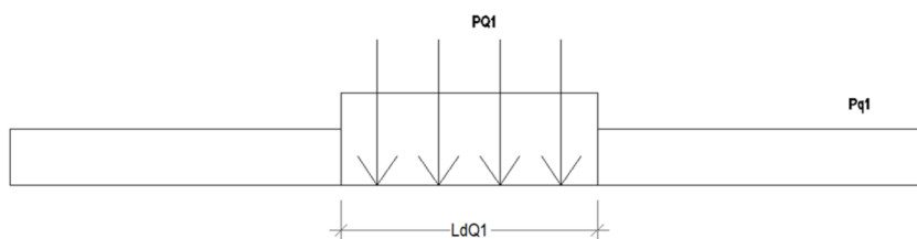
Figura 10. Carichi Treno LM71 su Ld
