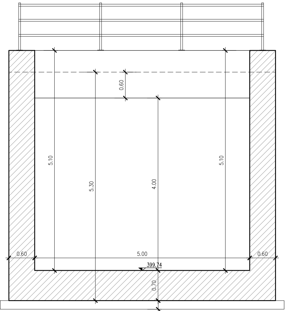
SEZIONE 1-1 Scala 1:50
