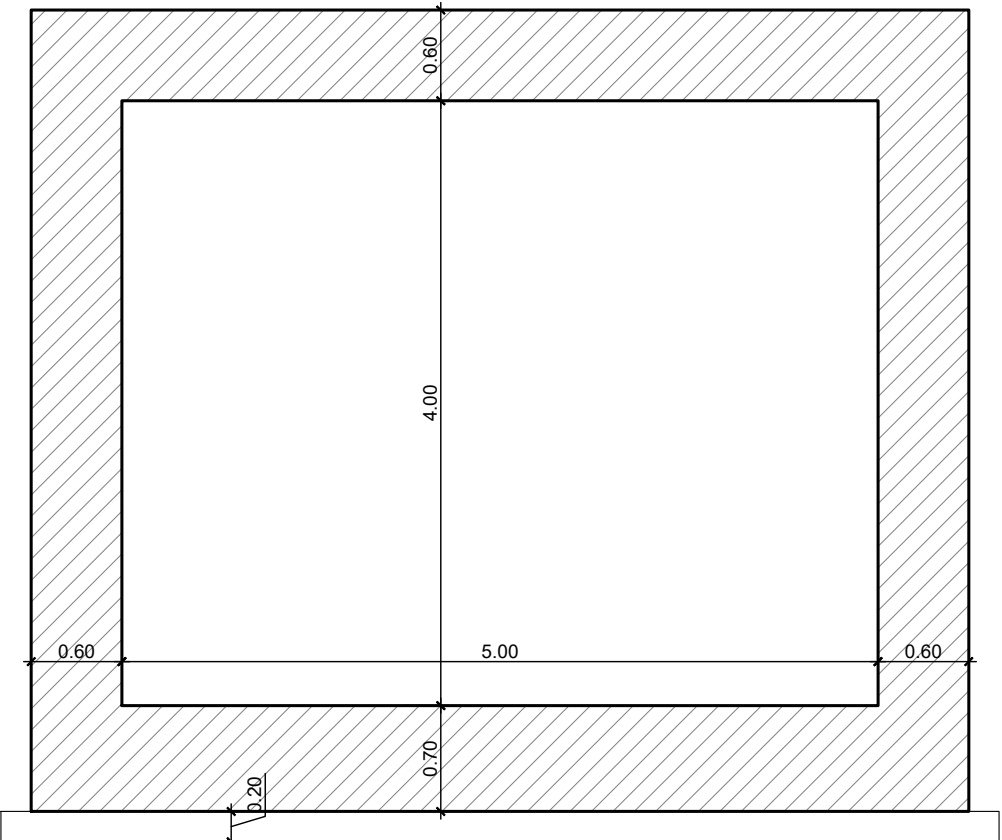
SEZIONE 2-2 Scala 1:50
