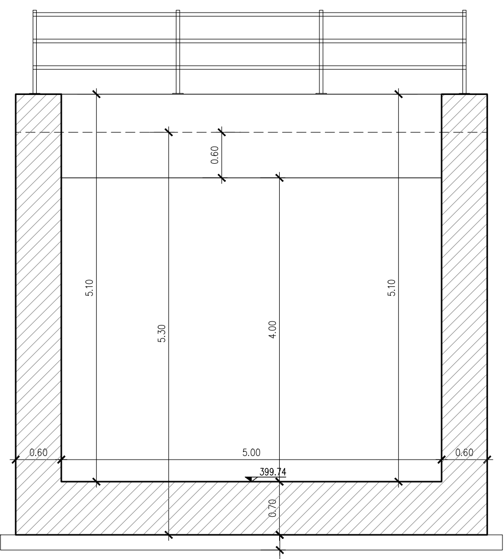
SEZIONE 3-3 Scala 1:50
