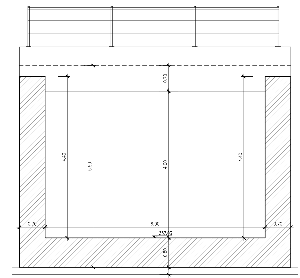
SEZIONE 1-1 Scala 1:50
