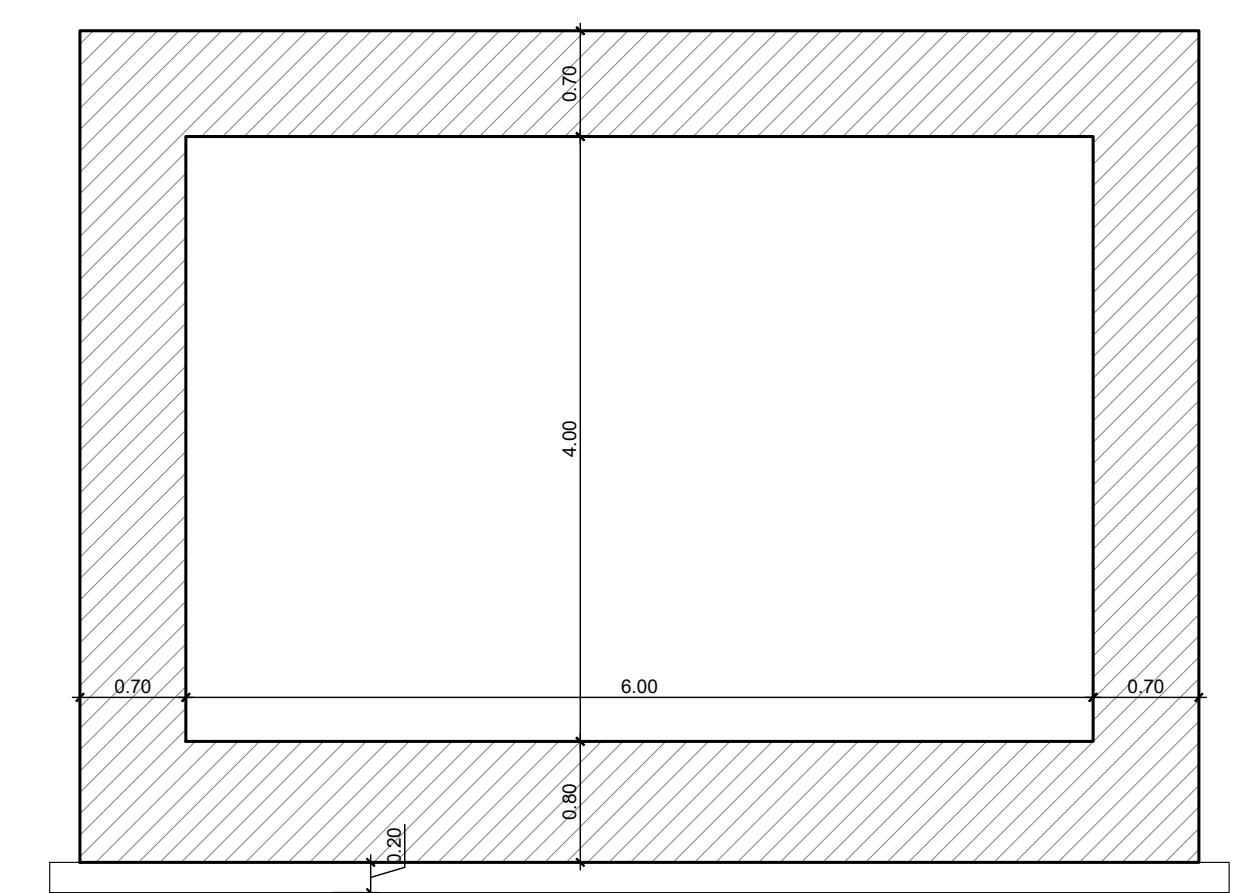
SEZIONE 2-2 Scala 1:50
