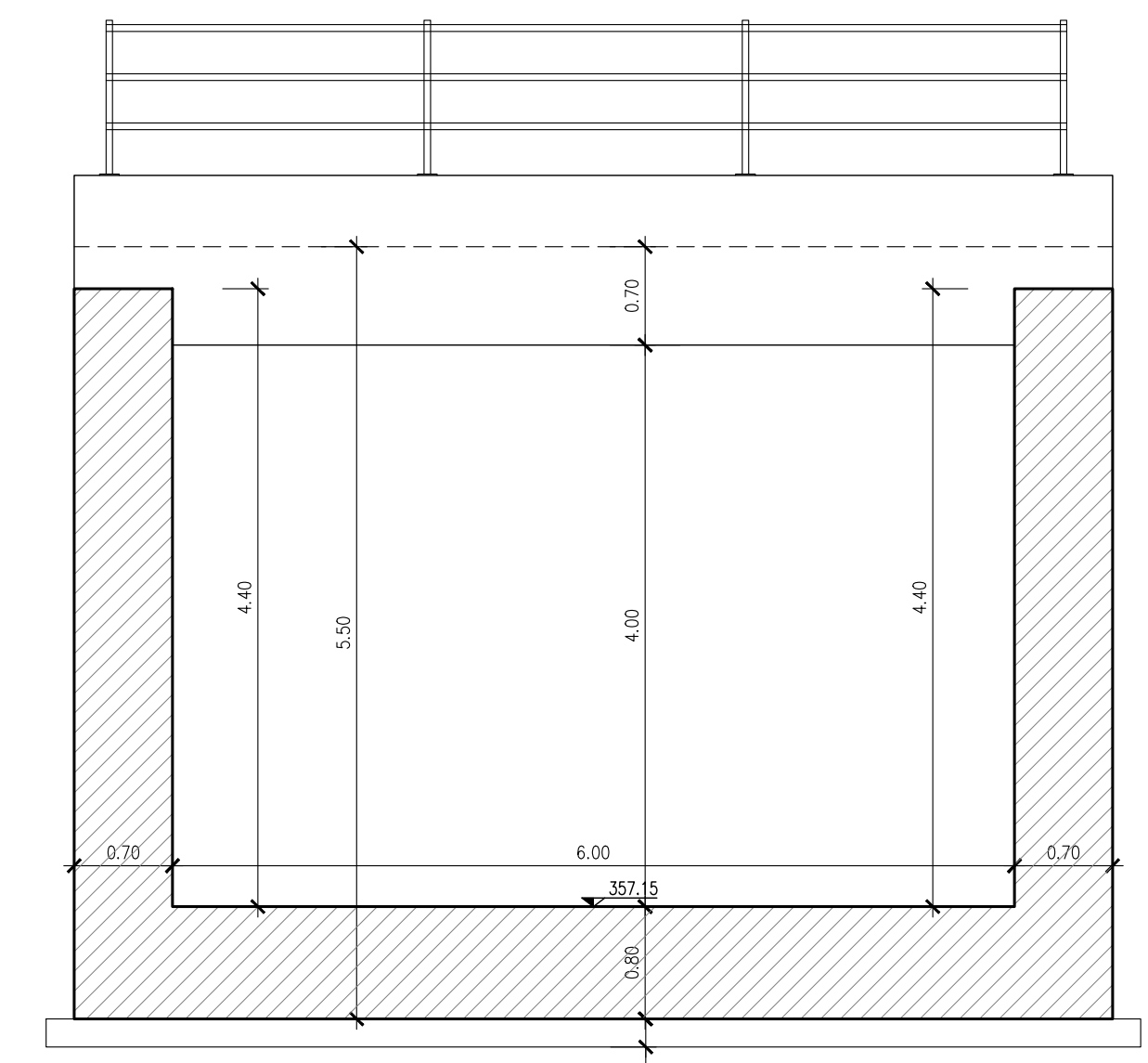
SEZIONE 3-3 Scala 1:50
