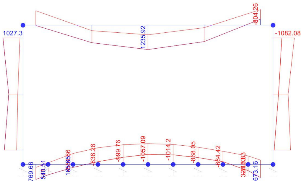
Momento Flettente
