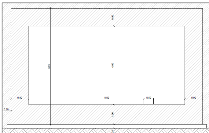
Figura 1c. Sezione trasversale dello scatolare
