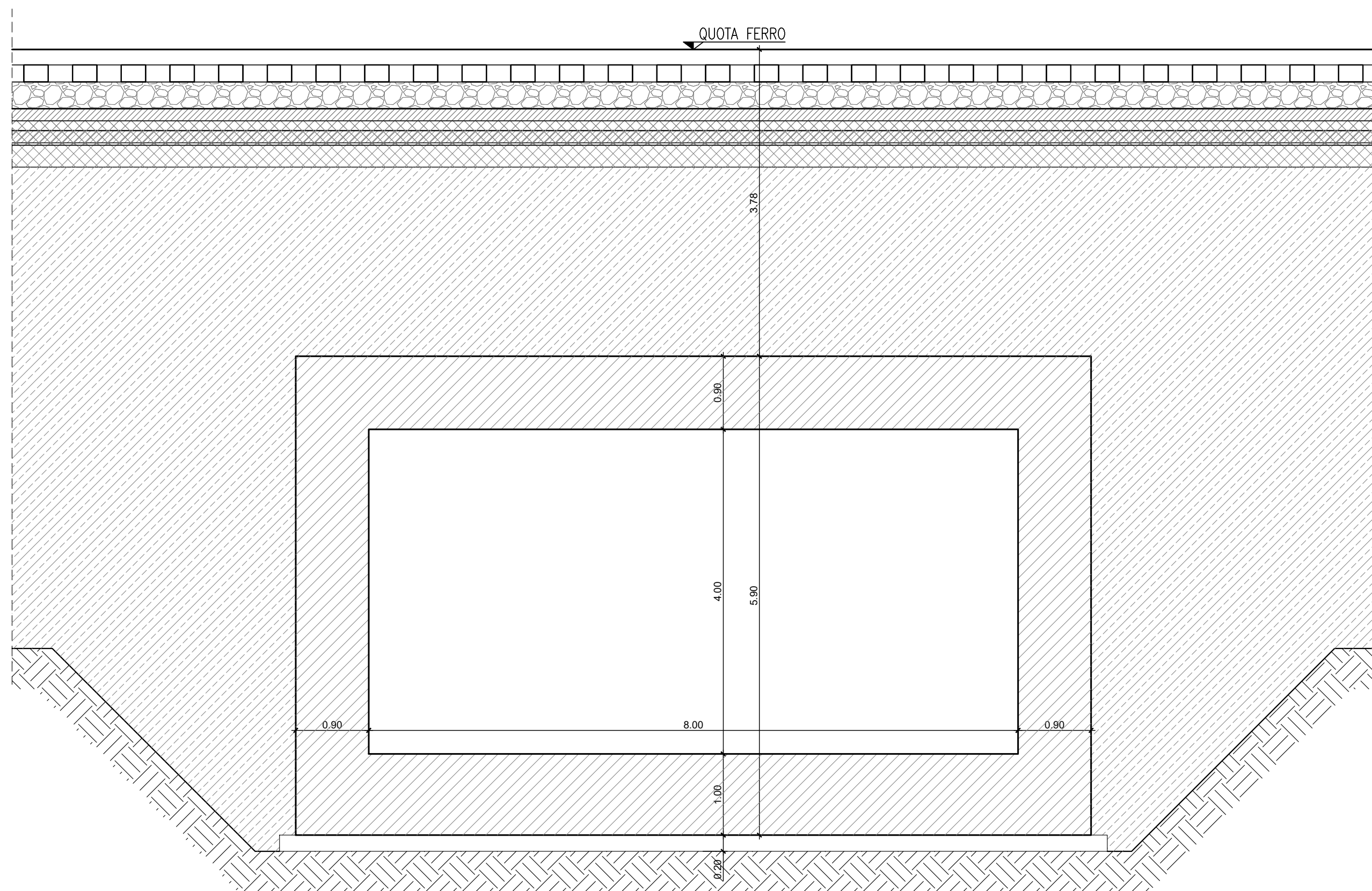
Tombino scatolare 8x4 Sezione su BP LV Scala 1:50
