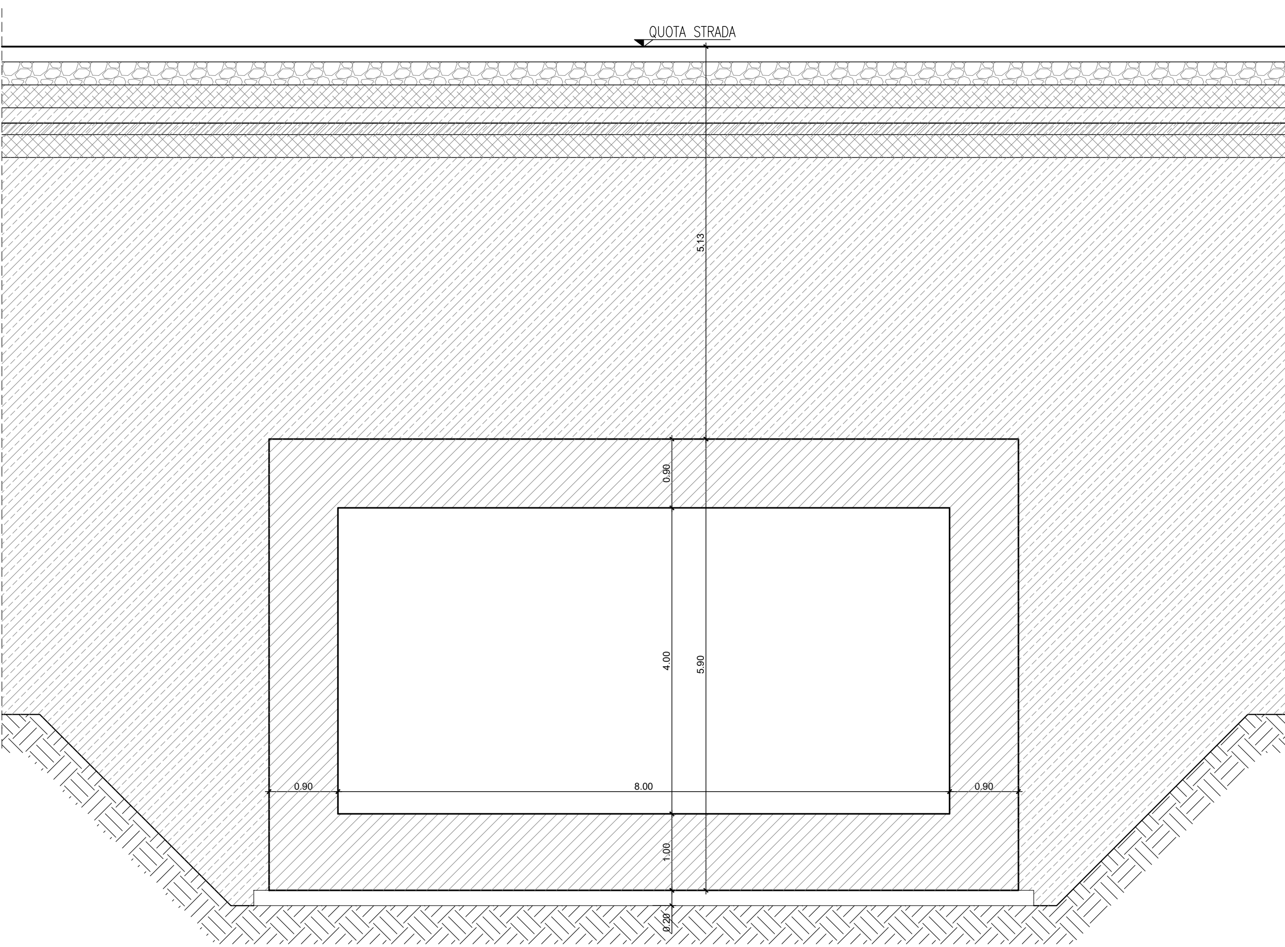
Tombino scatolare 8x4 Sezione su NV98 Scala 1:50
