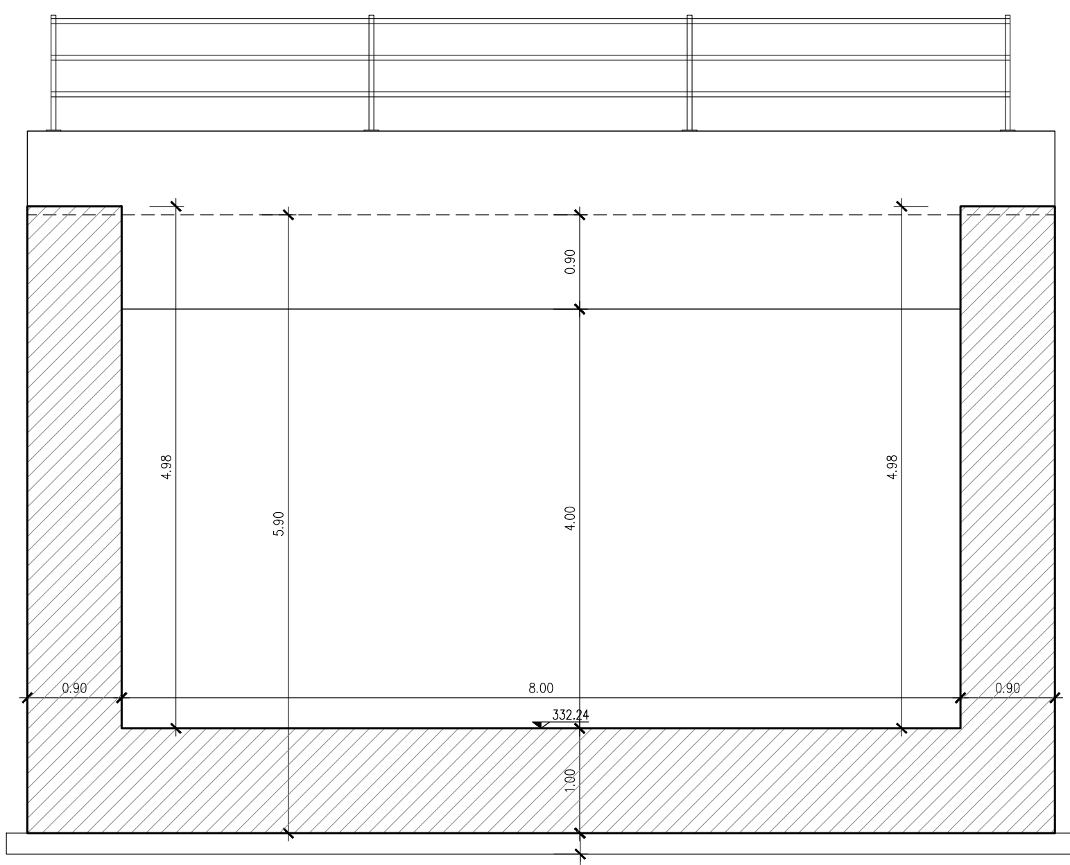
SEZIONE 3-3 Scala 1:50
