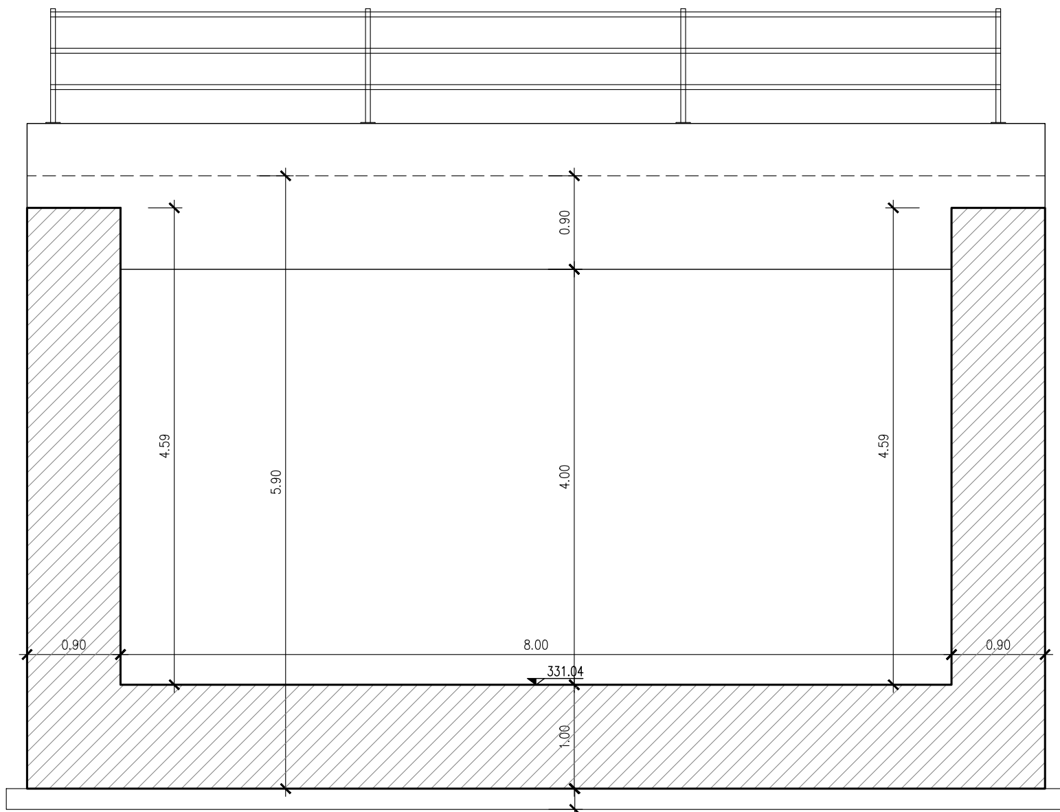
SEZIONE 1-1 Scala 1:50
