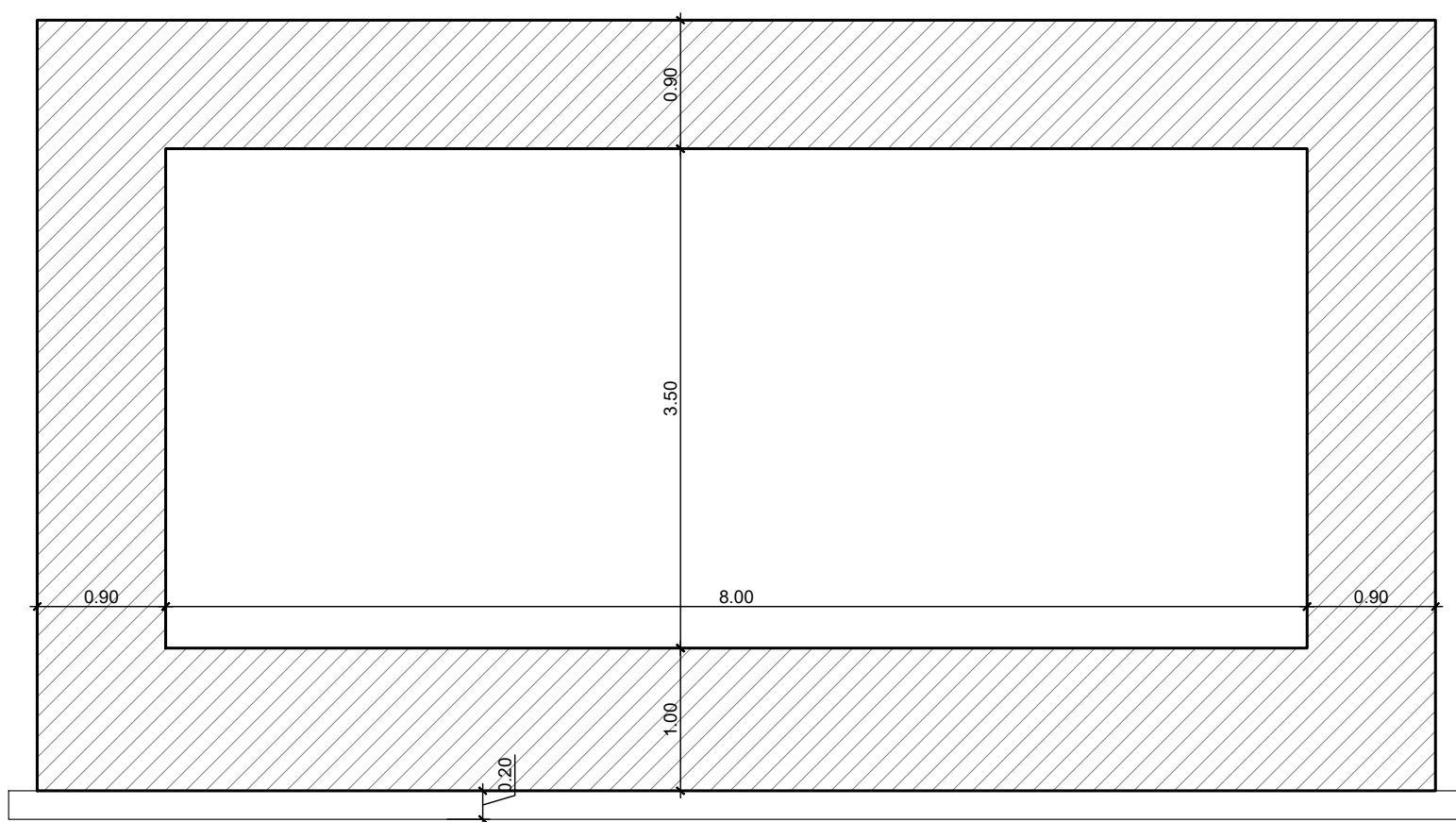
SEZIONE 2-2 Scala 1:50
