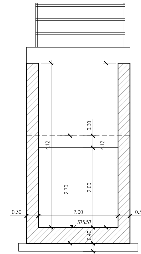
SEZIONE 1-1 Scala 1:50
