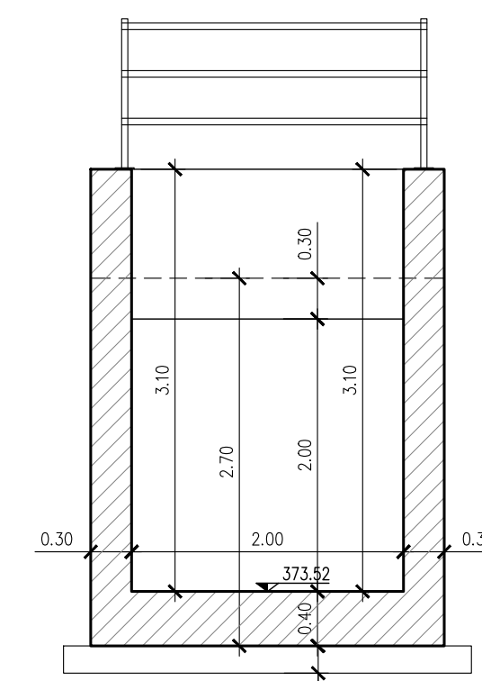
SEZIONE 3-3 Scala 1:50
