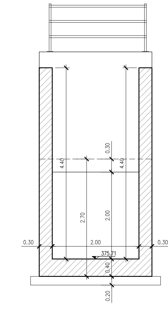
SEZIONE 3-3 Scala 1:50
