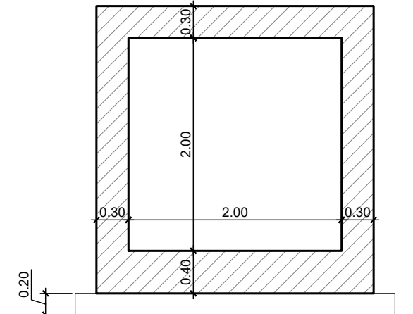
SEZIONE 2-2 Scala 1:50
