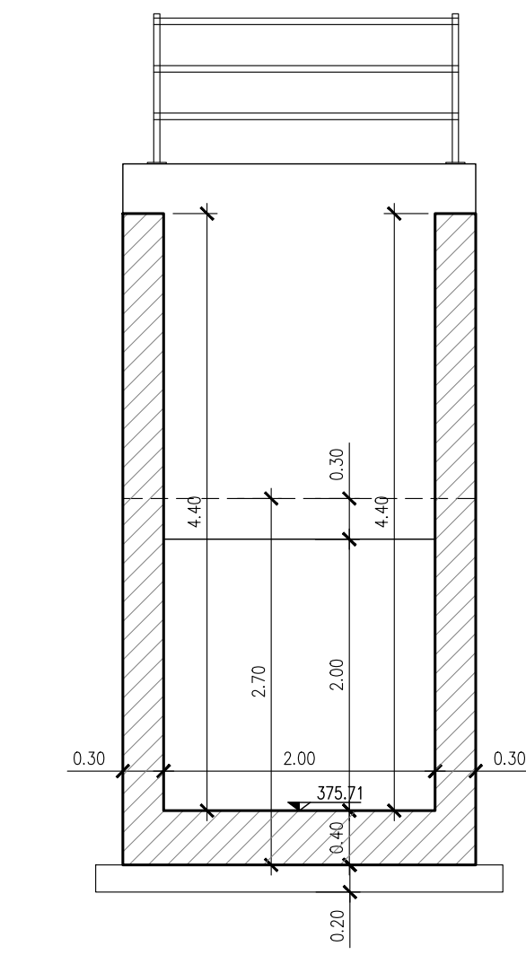
SEZIONE 1-1 Scala 1:50
