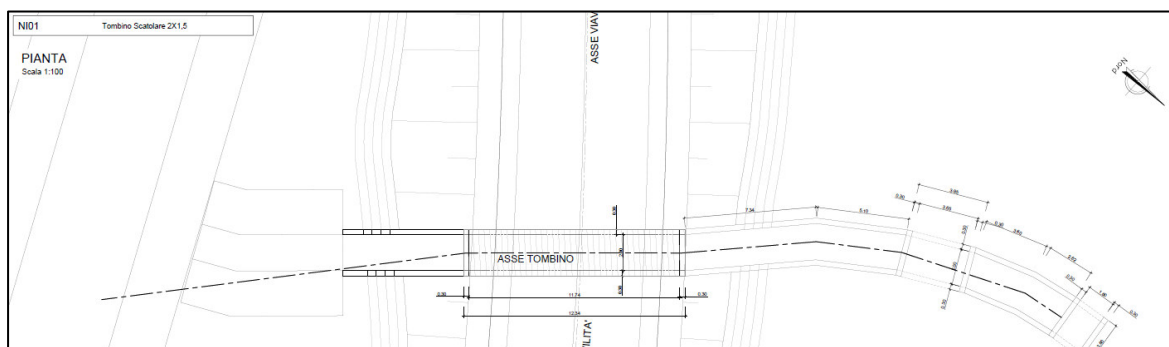
Figura 1a. Stralcio planimetrico dello scatolare
