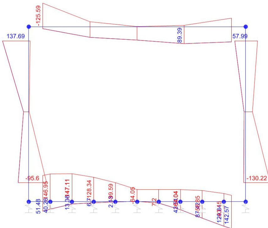
Momento Flettente
