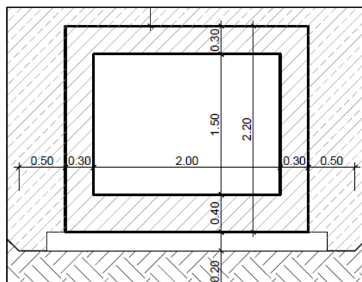
Figura 1c. Sezione trasversale dello scatolare
