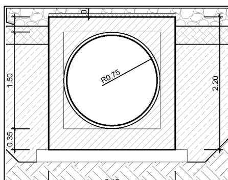
Figura 1c. Sezione trasversale dello scatolare
