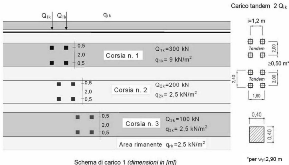
Figura 7 – Schema di Carico 1 del D.M. 17/01/2018
