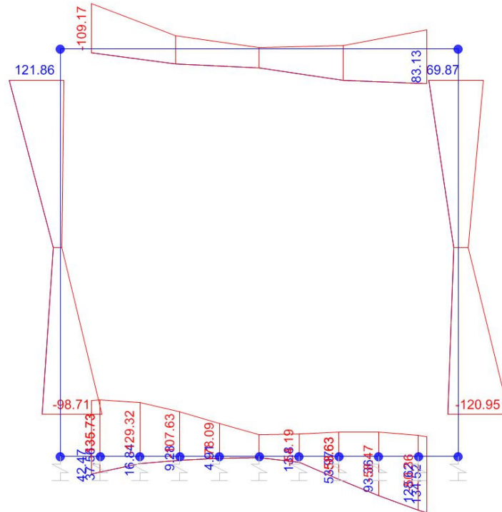
Momento Flettente
