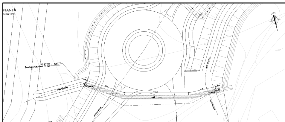
Figura 1a. Stralcio planimetrico dello scatolare
