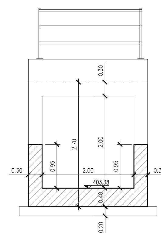
SEZIONE 1-1 Scala 1:50
