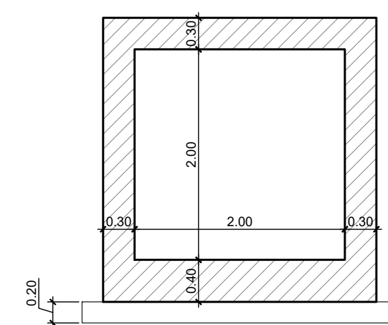
SEZIONE 2-2 Scala 1:50
