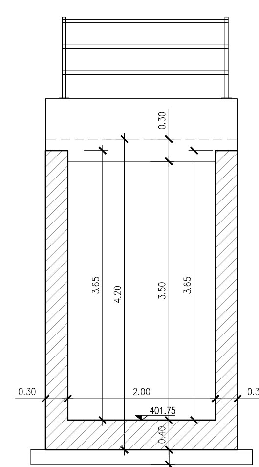
SEZIONE 3-3 Scala 1:50
