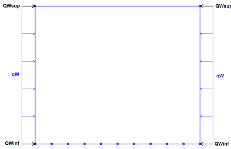
Figura 13. Condizione di carico SPSDX e SPSSX da SAP2000
