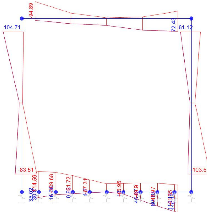
Momento Flettente
