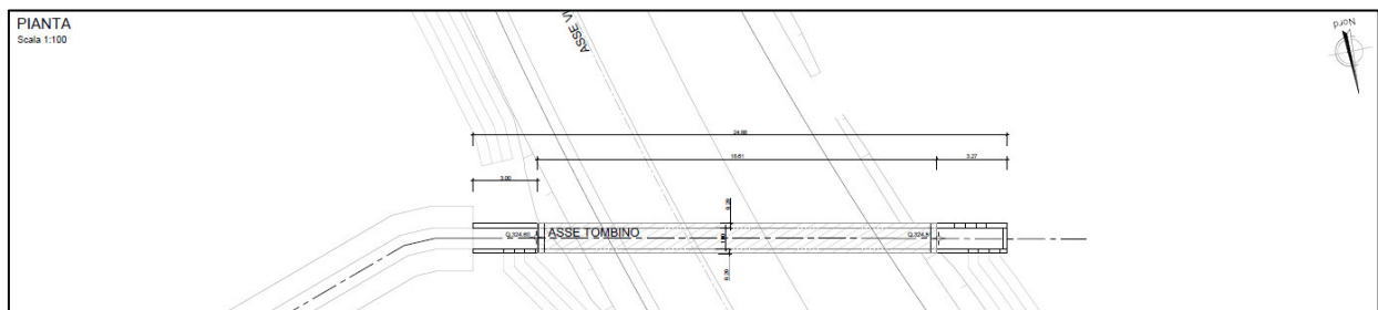
Figura 1a. Stralcio planimetrico dello scatolare
