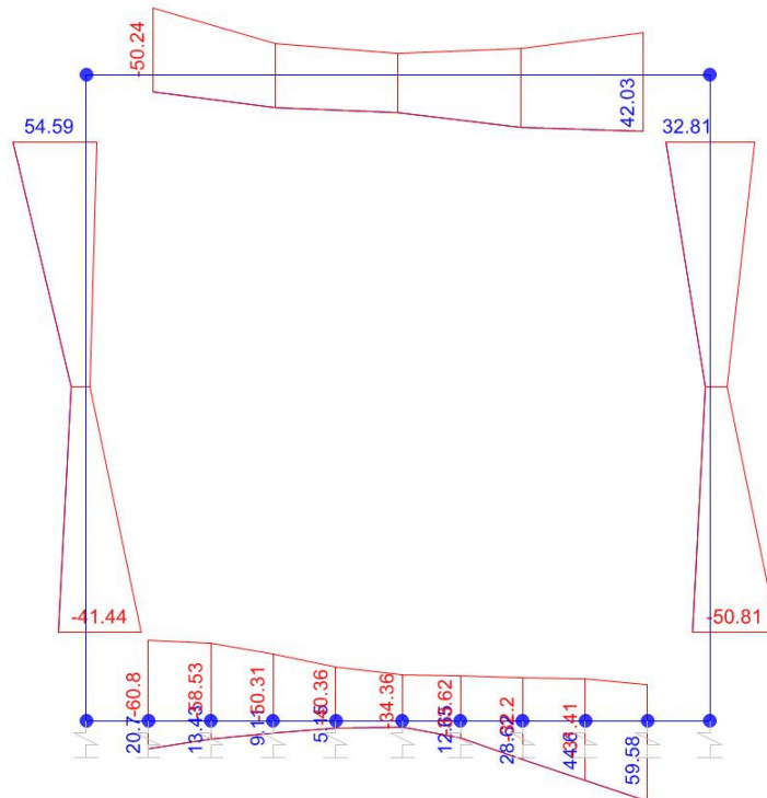
Momento Flettente
