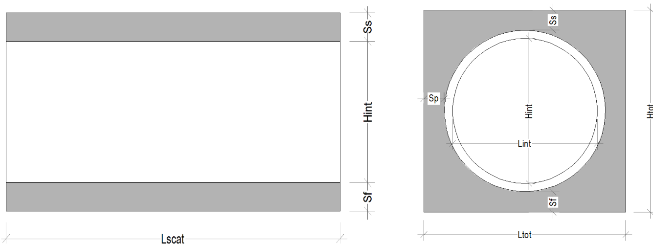
Figura 2. Simbologia adottata
