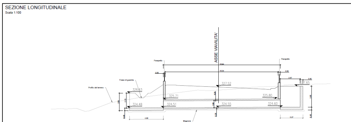
Figura 1b. Sezione longitudinale dello scatolare
