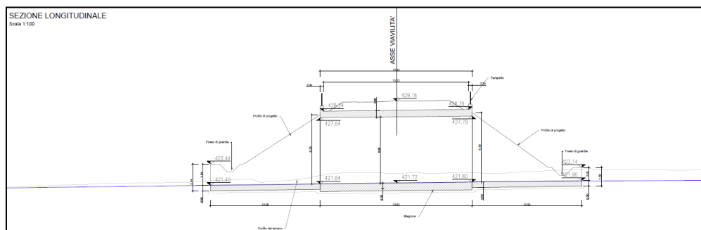
Figura 1b. Sezione longitudinale dello scatolare
