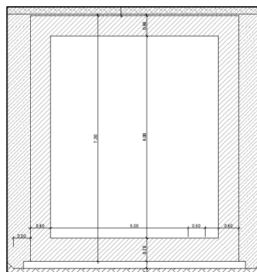
Figura 1c. Sezione trasversale dello scatolare
