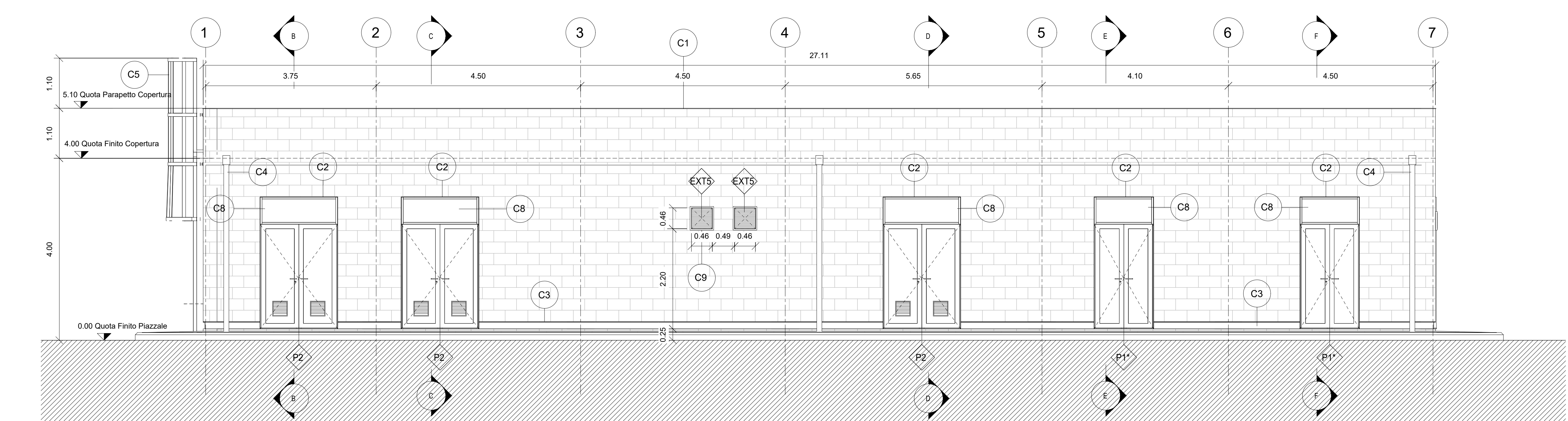
Prospetto P3 1:50
