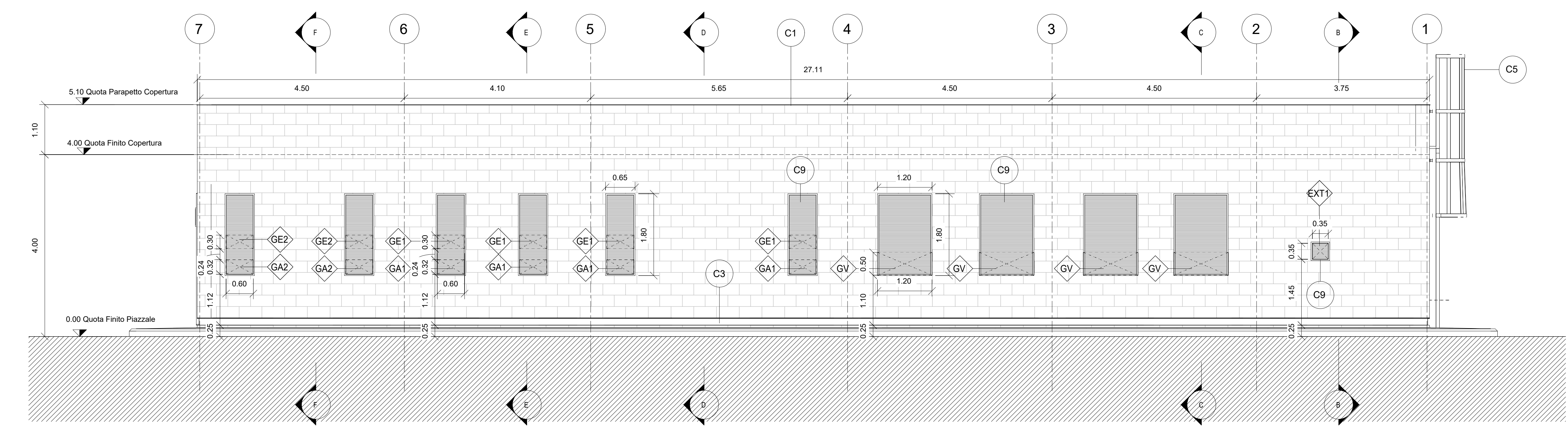
Prospetto P1 1:50
