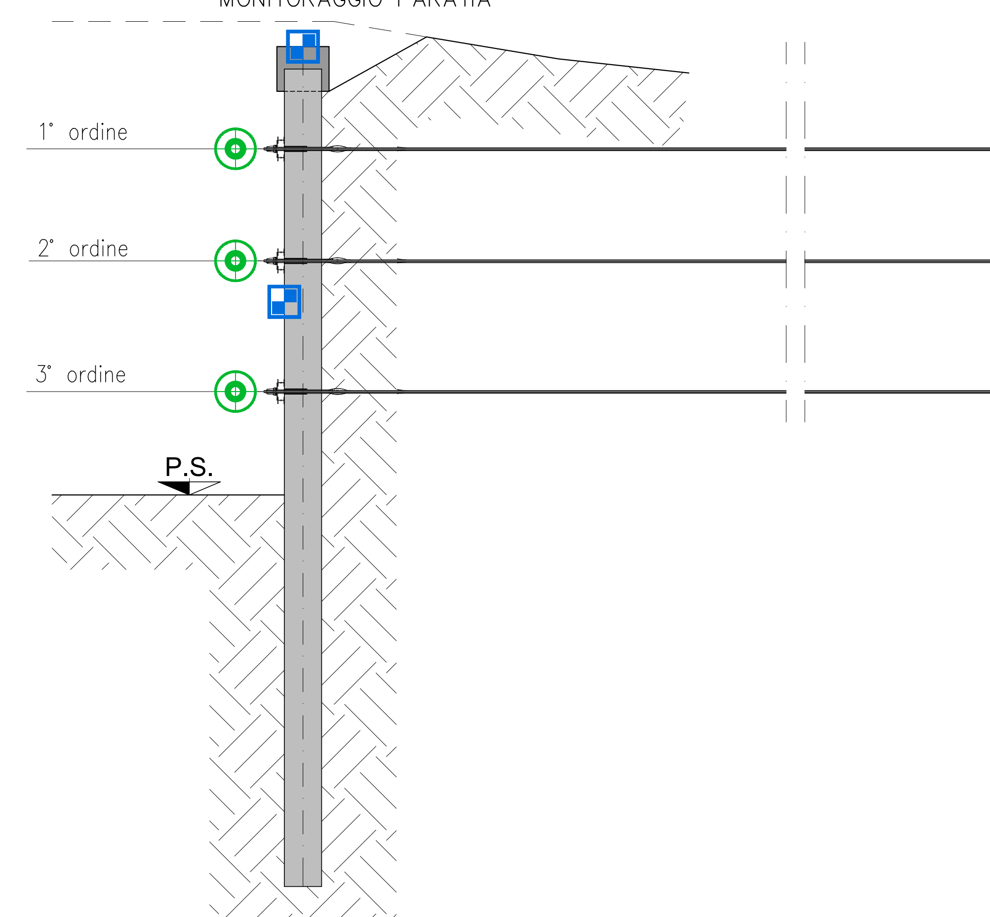
SEZIONE A-A SCALA 1:100 MONITORAGGIO PARATIA
