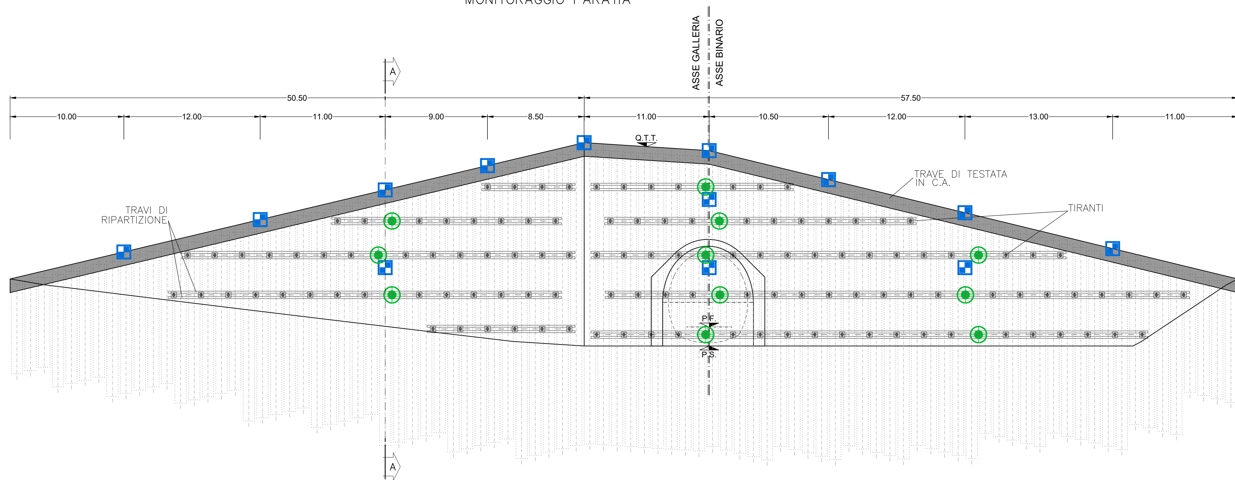
SVILUPPATA IN ASSE PARATIA SCALA 1:200 MONITORAGGIO PARATIA
