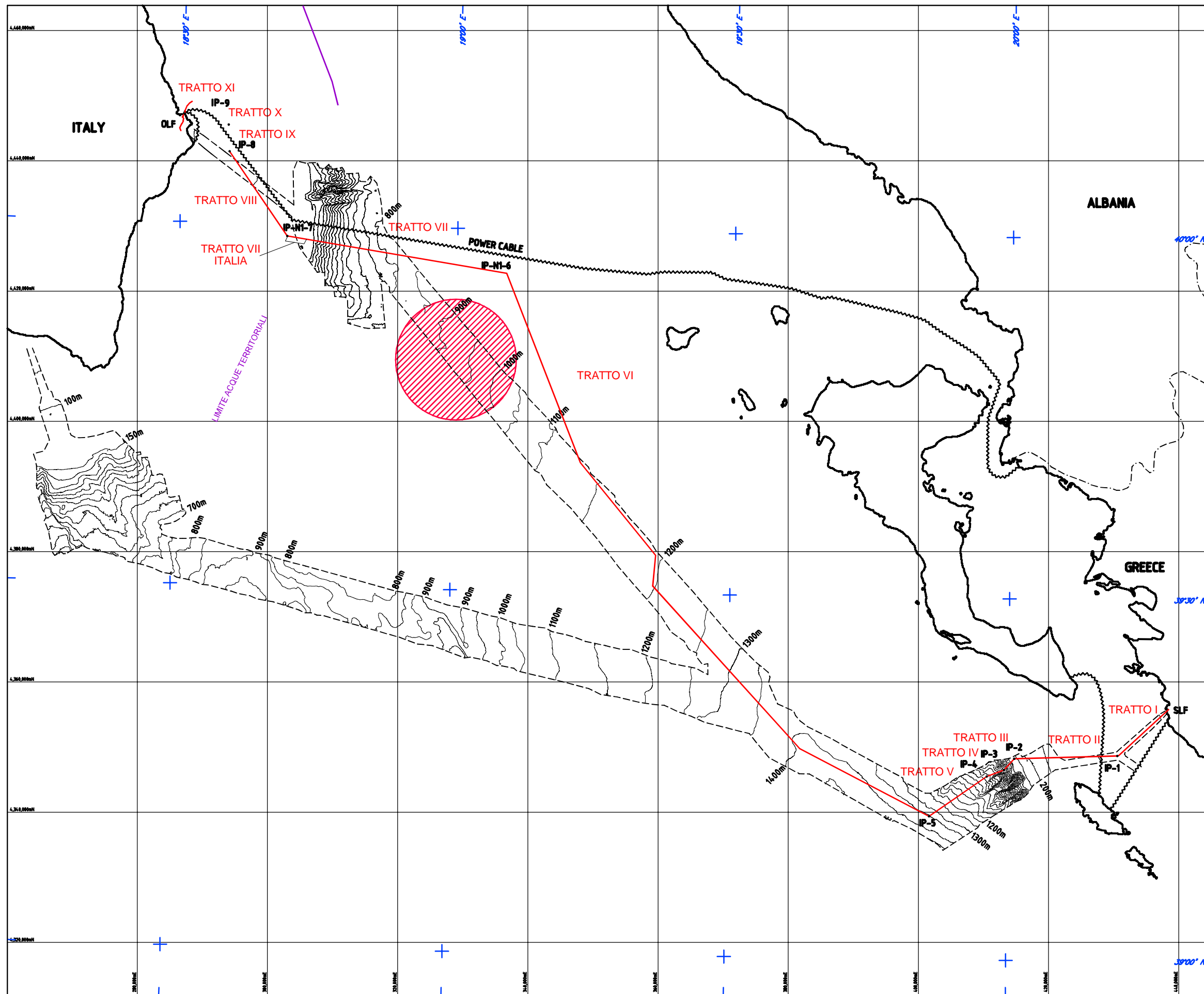
FIGURA 3.3 METANODOTTO DI INTERCONNESSIONE ITALIA - GRECIA TRACCIATO OFF-SHORE
