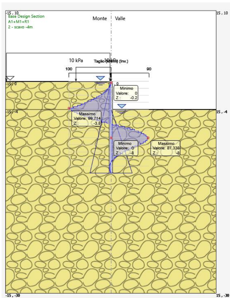
Figura 3: forza di taglio allo SLU-STR
