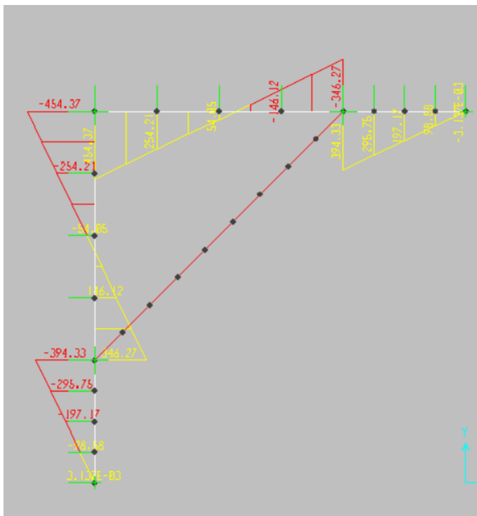
Figura 8: forza di taglio allo SLU-STR
