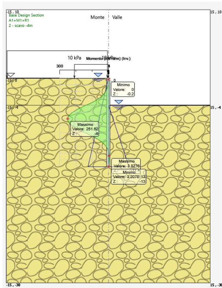
Figura 2: momento flettente allo SLU-STR
