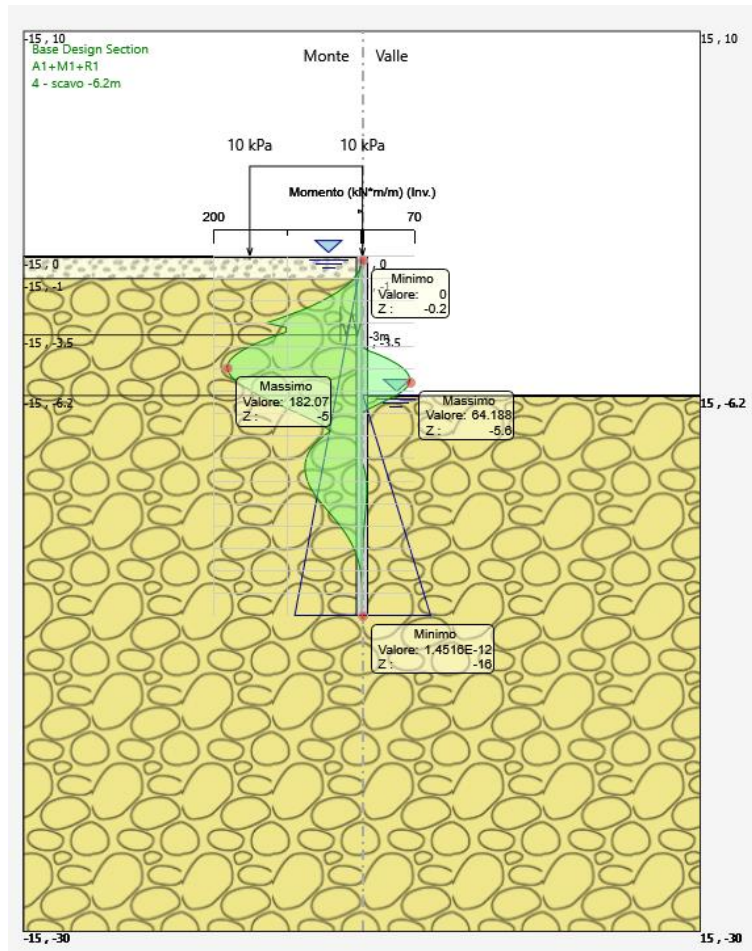
Figura 4: momento flettente allo SLU-STR
