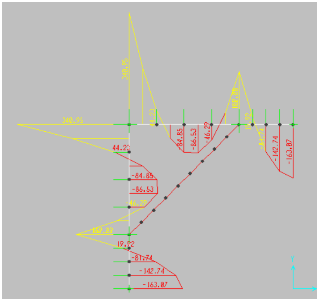
Figura 6: momento flettente allo SLU-STR
