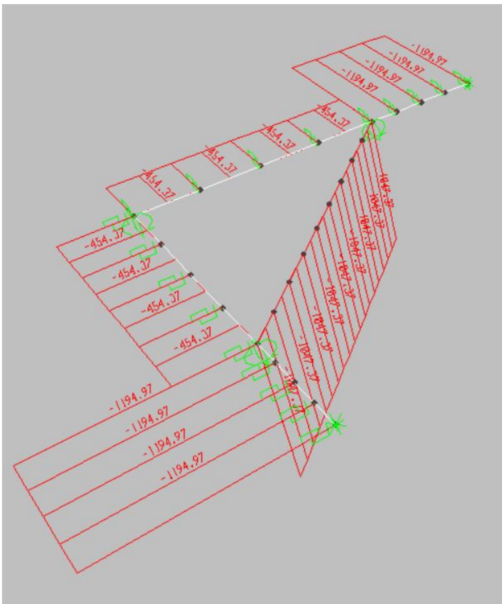
Figura 7: forza assiale allo SLU-STR
