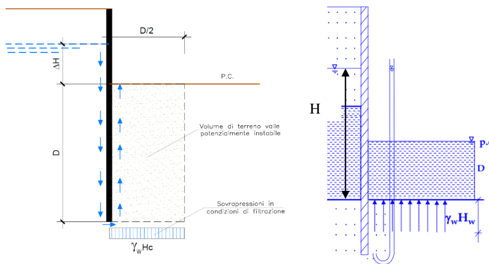
Figura 9: Schema di filtrazione per effetto di scavi sotto falda a valle di opere di sostegno
