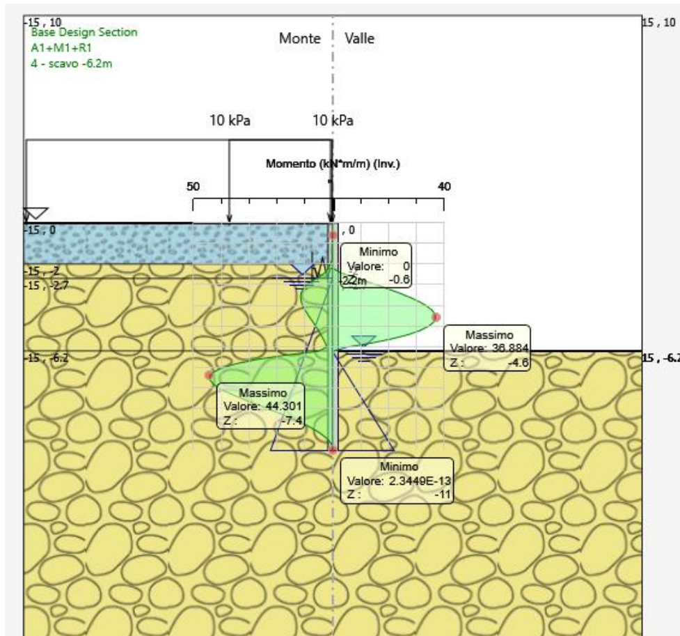
Figura 2: momento flettente allo SLU-STR
