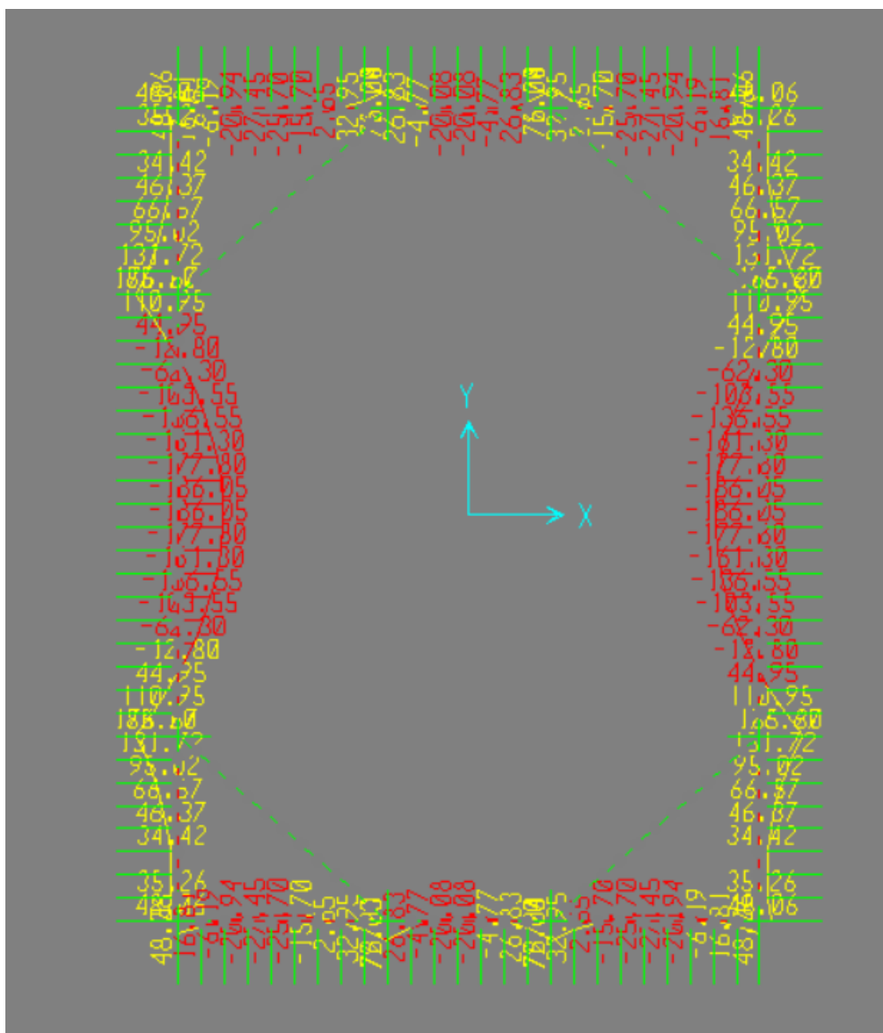
Figura 6: momento flettente allo SLU-STR
