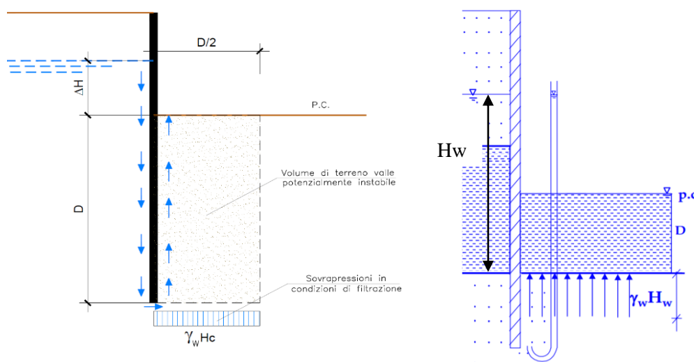
Figura 9: Schema di filtrazione per effetto di scavi sotto falda a valle di opere di sostegno
