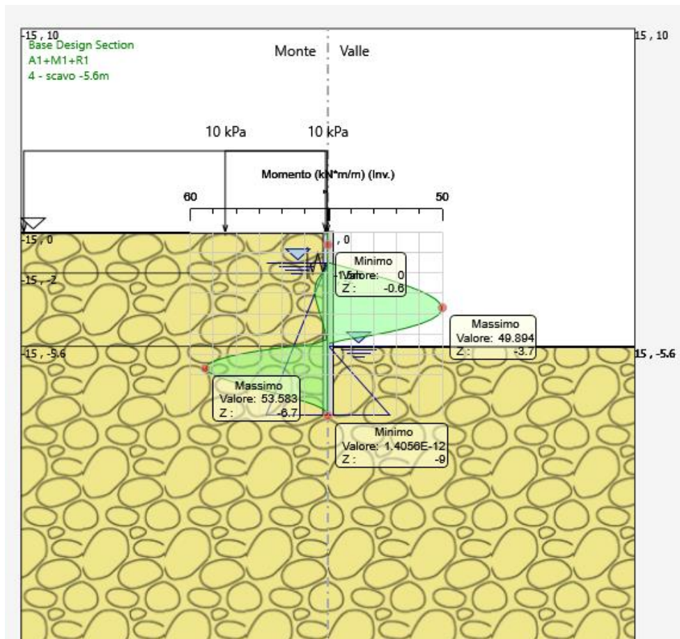
Figura 4: momento flettente allo SLU-STR
