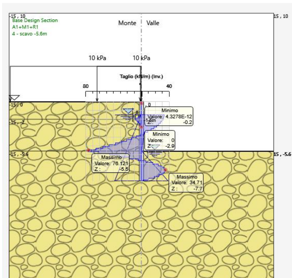
Figura 5: forza di taglio allo SLU-STR
