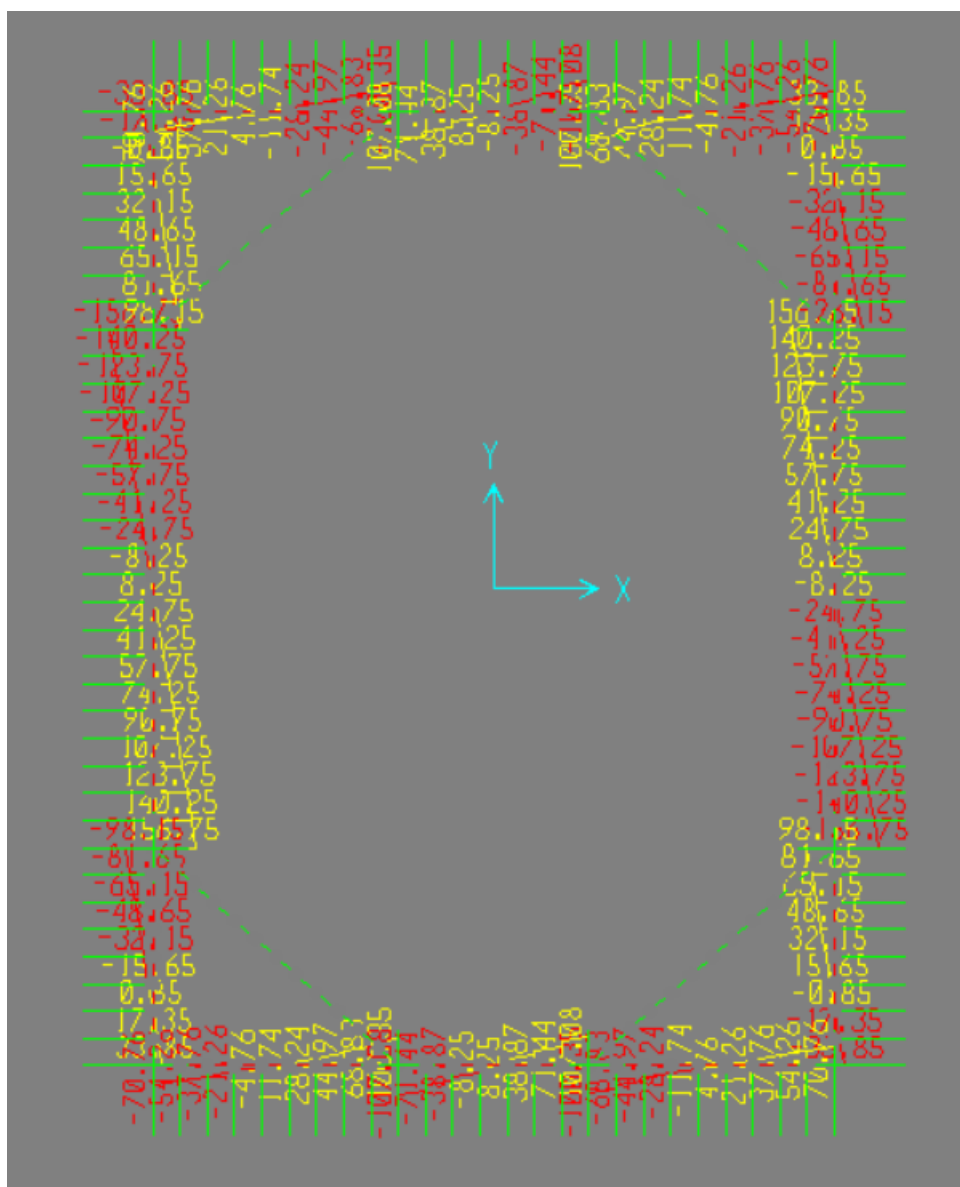
Figura 8: forza di taglio allo SLU-STR
