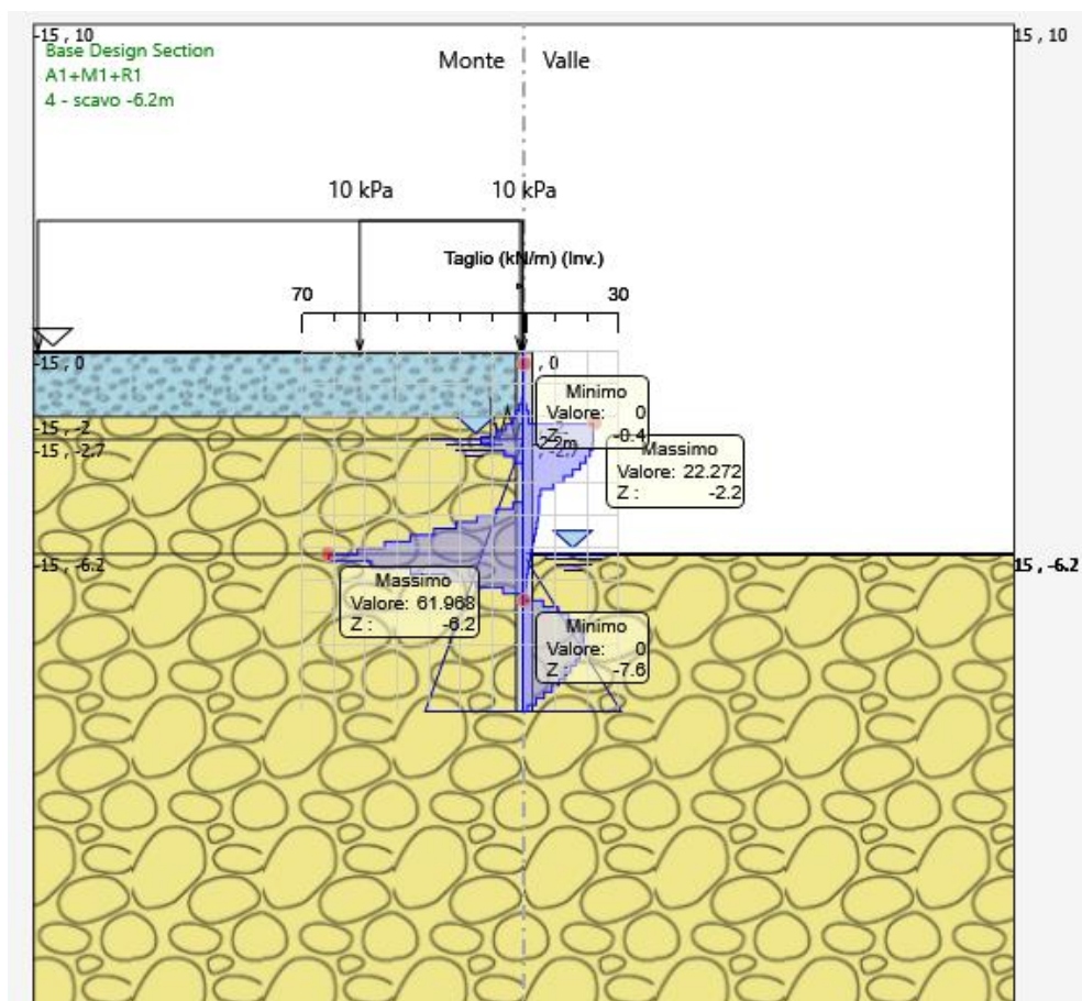
Figura 3: forza di taglio allo SLU-STR
